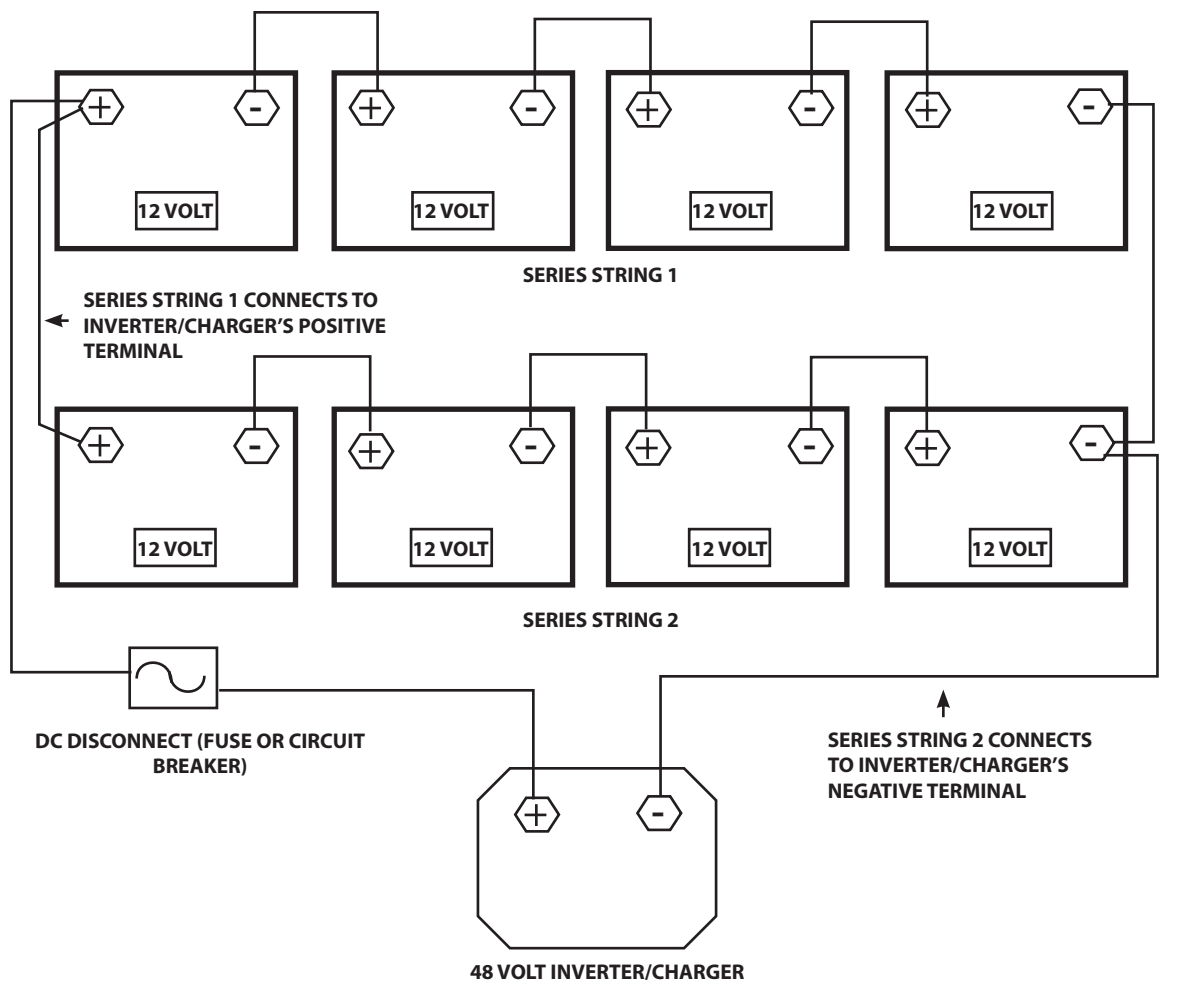
SERIES/PARALLEL/48 VOLT FX
