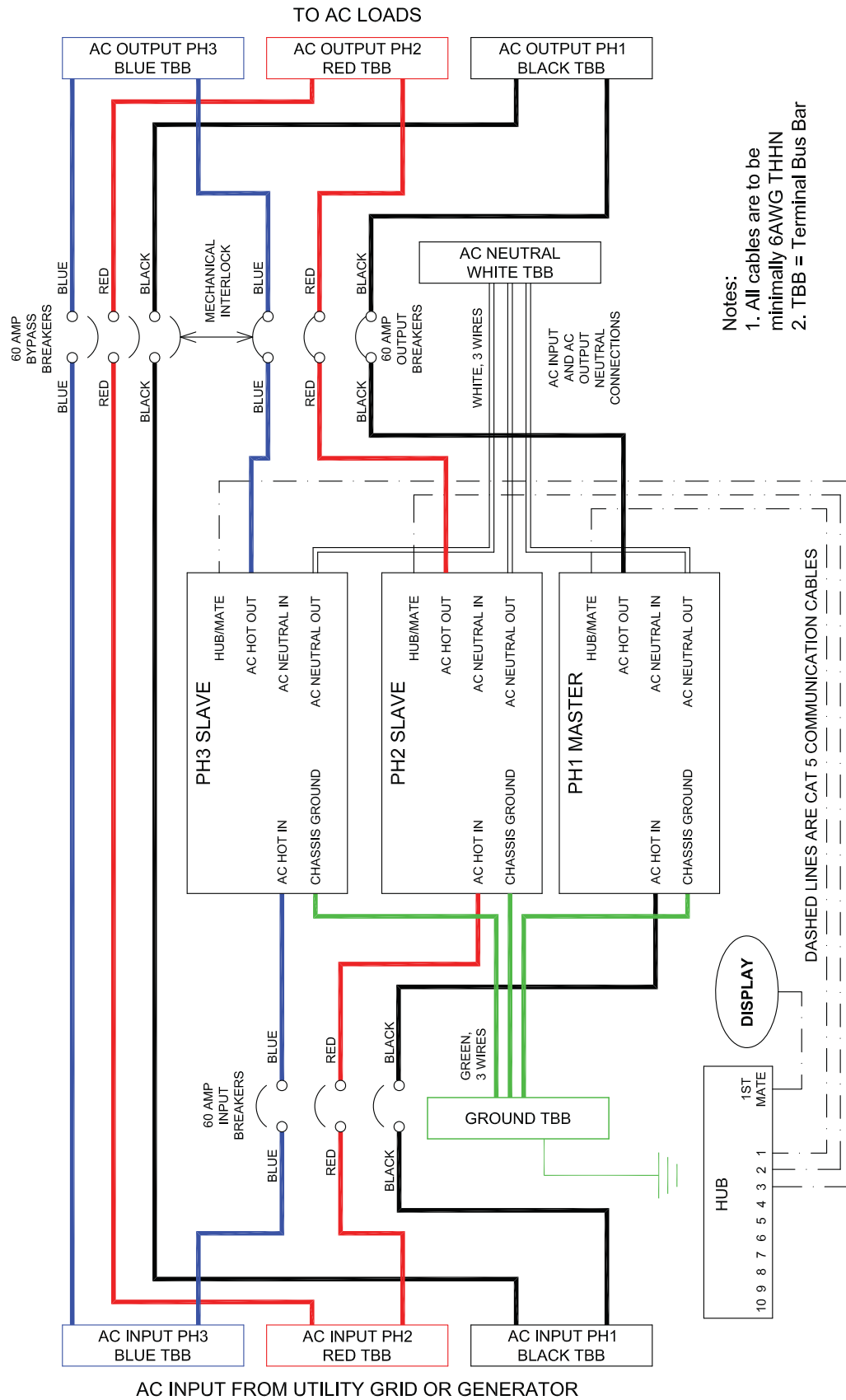
Sistema trifásico
