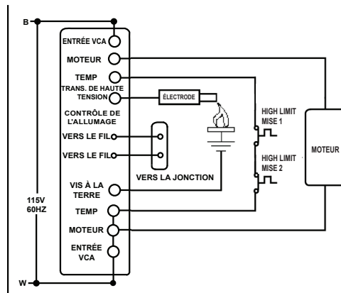
DIAGRAMME SCHEMATIQUE
