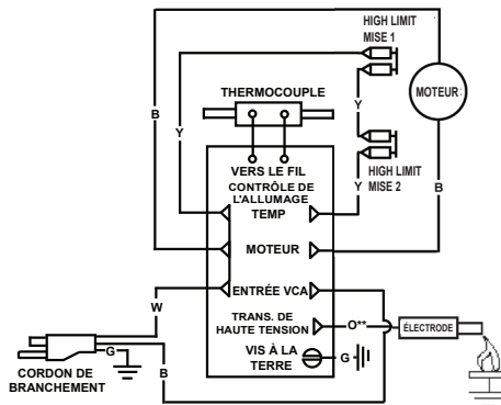
DIAGRAMME DE CONNEXION
