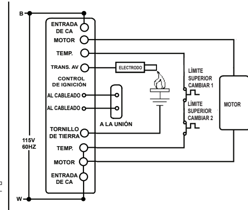
DIAGRAMA ESQUEMÁTICO
