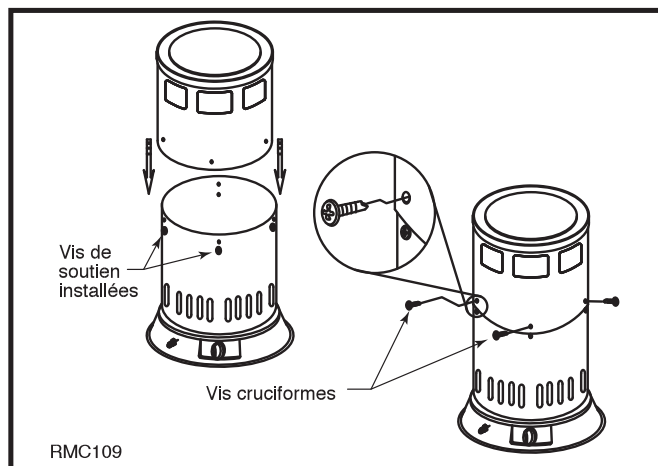
Schéma 4 : Fixez la partie supérieure du boîtier à l'aide de quatre vis cruciformes.
