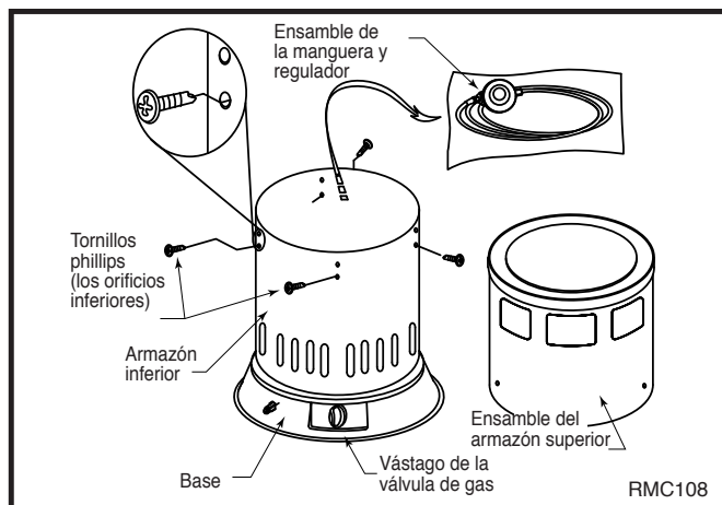
Fig. 3 Saque el conjunto de la manguera con regulador, coloque cuatro tornillos en los agujeros de la parte superior de la sección inferior de la carcasa.
