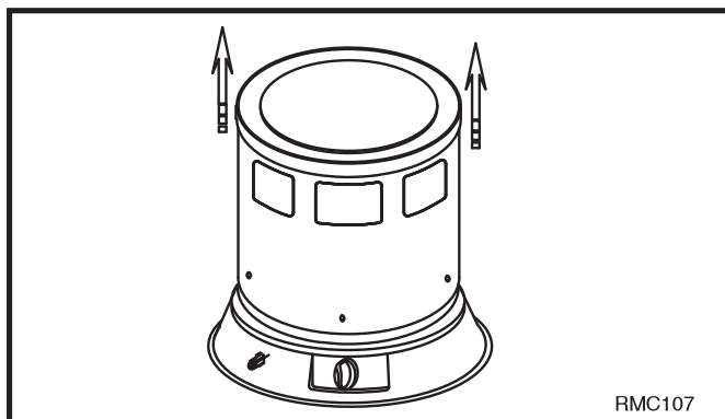
Schéma 2 : Faites glisser la partie supérieure du boîtier vers le haut pour la détacher de la partie inférieure.
