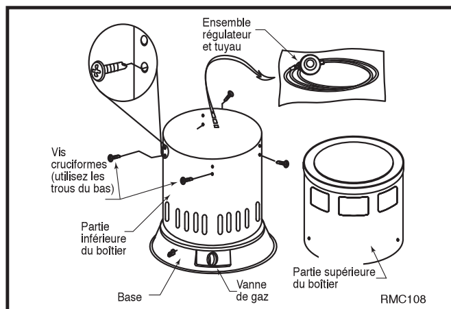
Schéma 3 : Retirez l'ensemble régulateur et tuyau et placez quatre vis dans les trous inférieurs situés au-dessus de la partie inférieure du boîtier.
