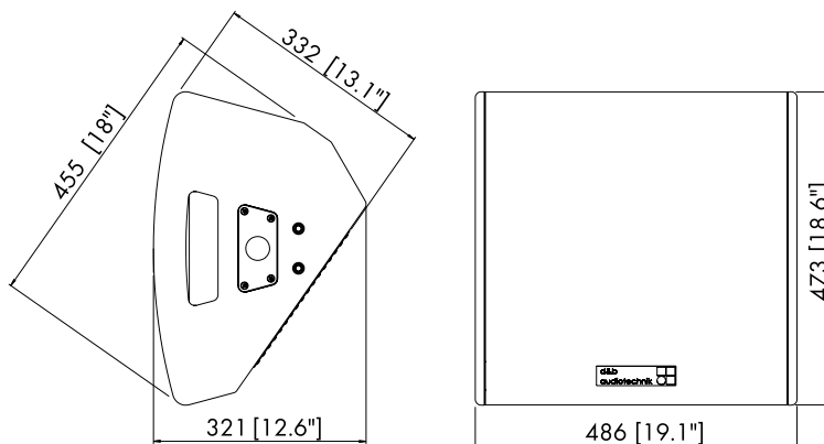
Dimensiones de la caja M6 en mm [pulg.]
