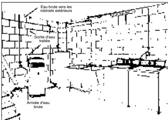
Installation de sous-sol type utilisant une tuyauterie suspendue avec orifice d'égout au sol ou cuve de buanderie à évacuation.
