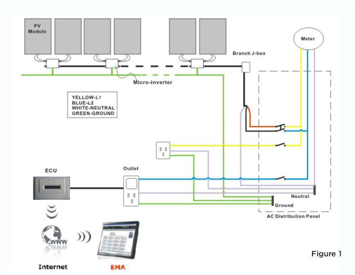
DIAGRAMA ESQUEMÁTICO DE INSTALACIÓN ELÉCTRICA
