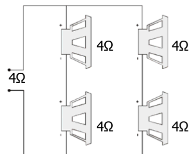
Conexión en serie/paralelo
