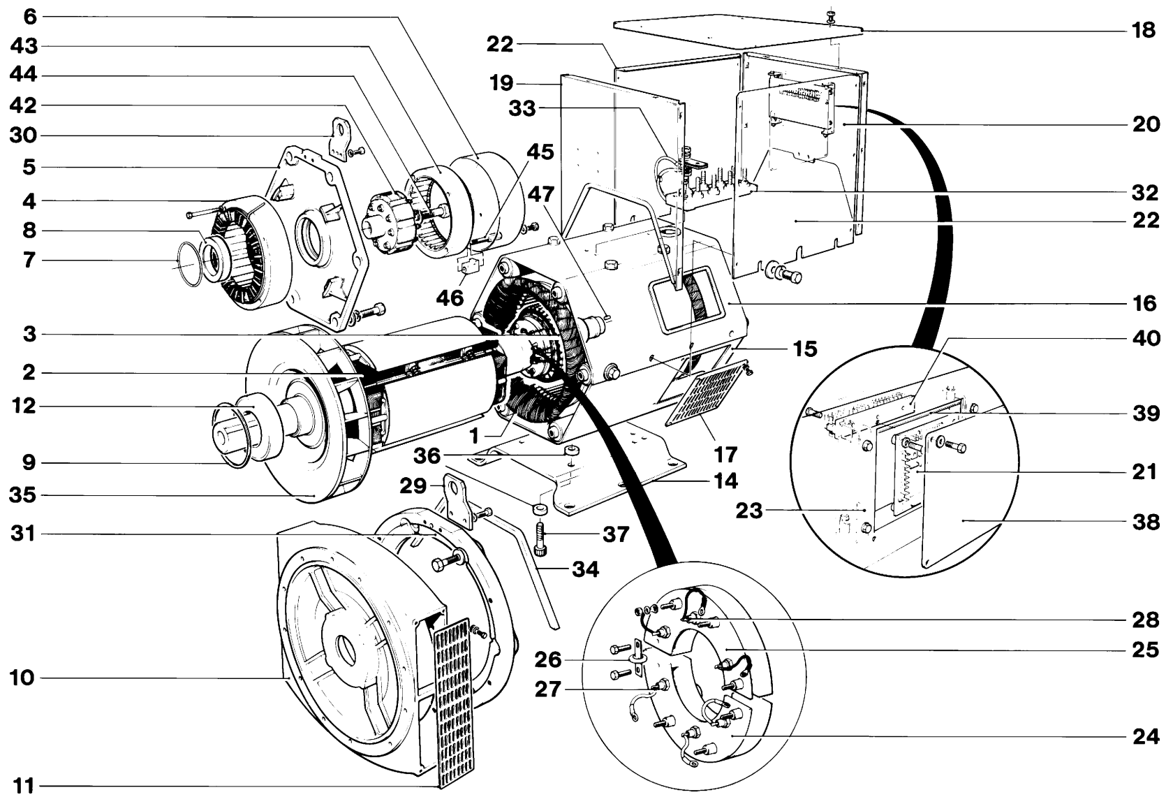
Fig. 12 GENERADOR TÍPICO DE DOS COJINETES
