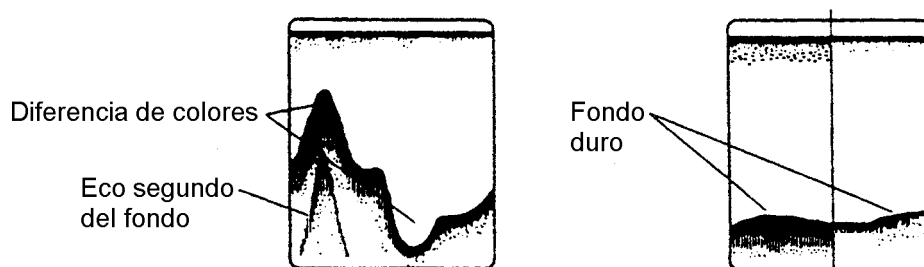
Perfil y material del fondo
