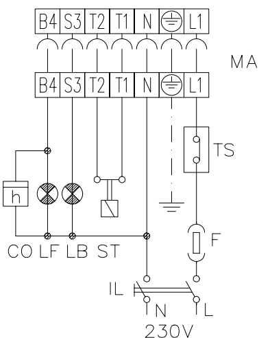
Fig. 7a - Quemadores de una etapa
