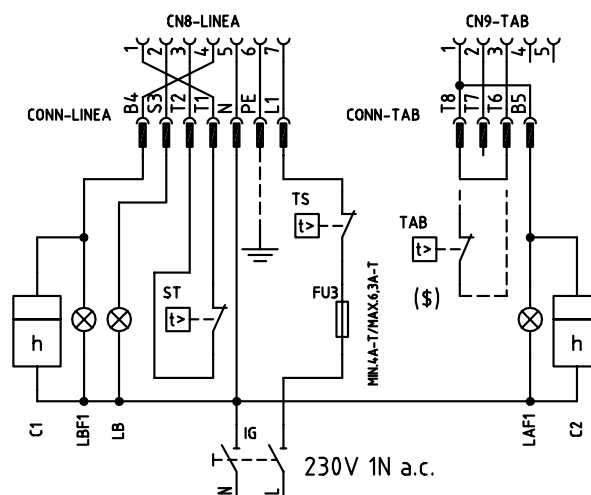
Fig. 7b - Quemadores de dos etapas
