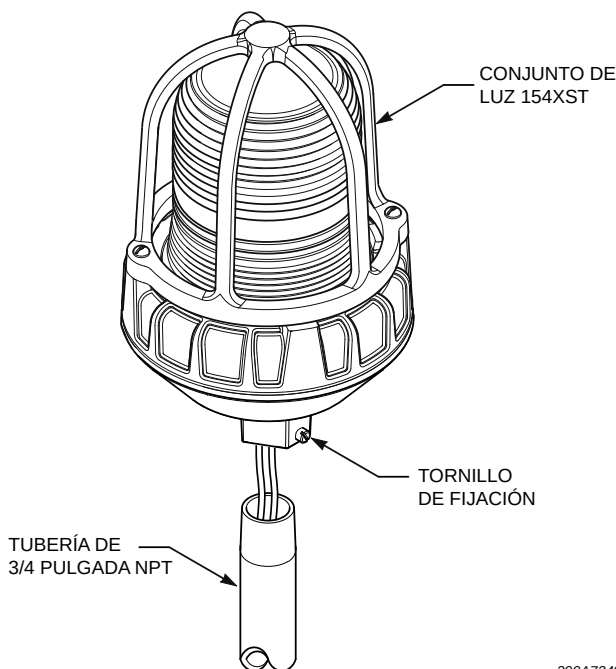
Figura 1 Baliza montada en una tubería
