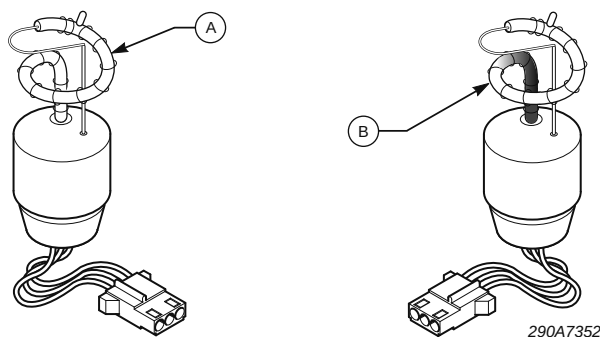
Figura 4 Oscurecimiento del tubo de intermitencia
