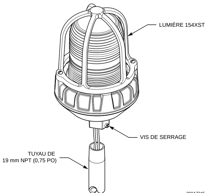
Figure 1 Lumière fixée sur un tuyau
