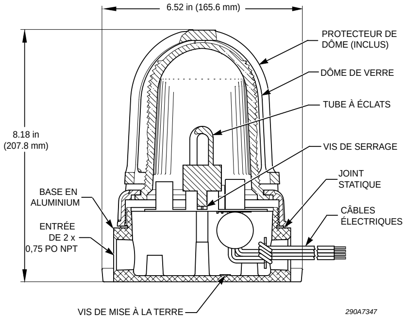
Figure 3 Coupe transversale de la lumière
