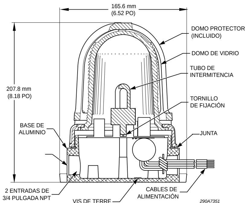
Figura 3 Corte transversal de la baliza
