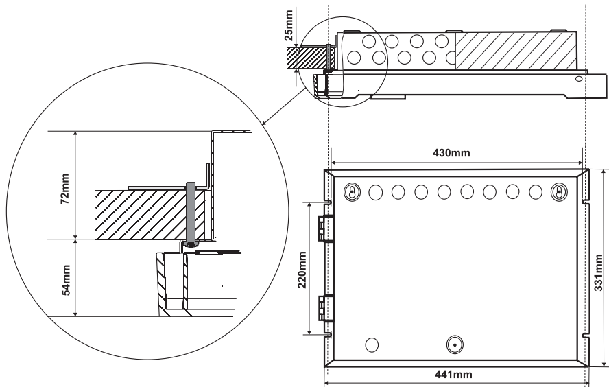
Figura 8. Agujeros de montaje empotrado. Vista principal de la fijación a los soportes de la pared y de los tornillos que soportan la caja metálica.
