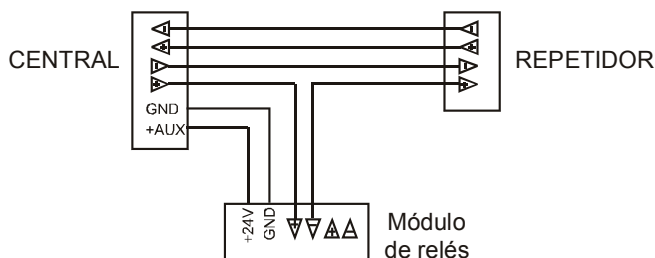
Figura 21. Conexión entre un Módulo de Relés, Repetidor y Central Maestra.
