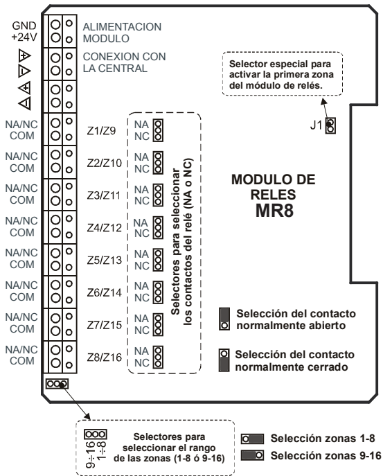
Figura 17. Configuración de terminales y puentes del MR8.
