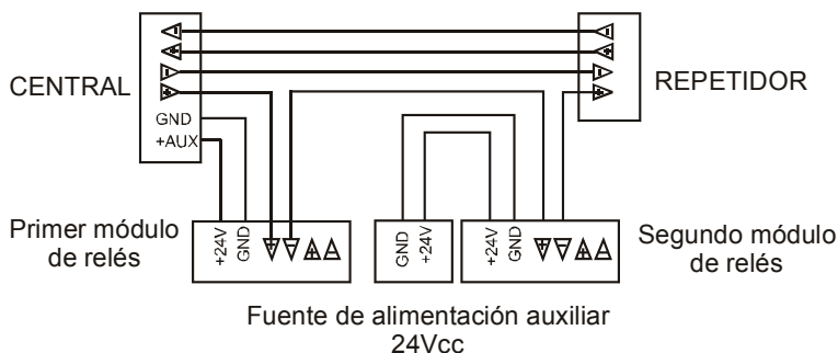
Figura 22. Conexión entre dos Módulos de Relés, Repetidor y el Central Maestra.
