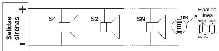
Figura 24. Conexión de sirenas a salidas SND1÷SND4 del módulo de control y a la salida de la tarjeta de 4 salidas de sirenas.
