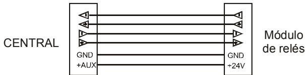
Figura 18. Conexión entre un Módulo de Relés y la Central.
