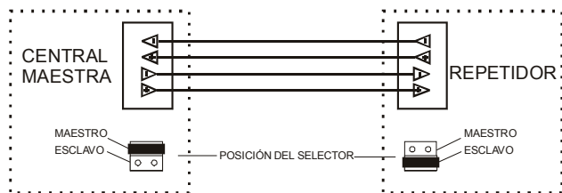
Figura 20. Conexión entre las Centrales Repetidor y Maestra.
