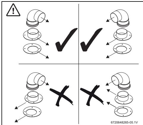
Fig. 11 Detalle de la instalación del collarín del kit AZ 219
