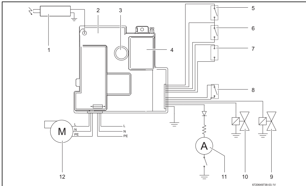
Fig. 3 Esquema eléctrico
