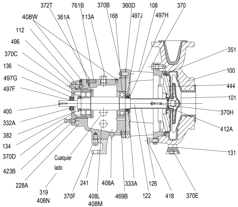
Imagen 61: Plano de la sección transversal del modelo 3198
