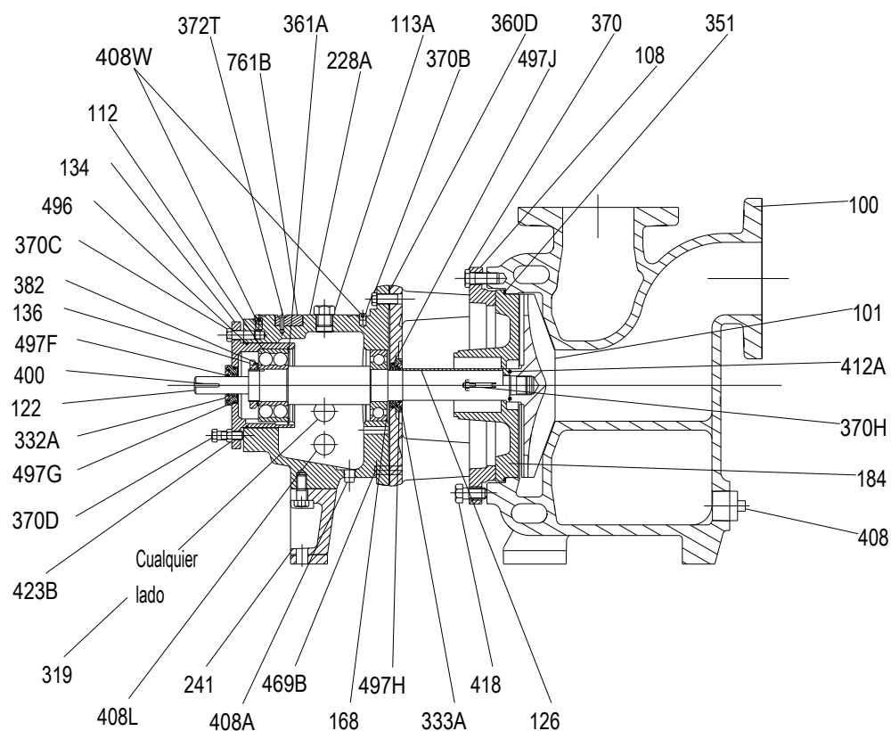
Imagen 62: Plano de la sección transversal del modelo 3796
