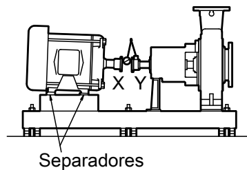
Imagen 23: Ejemplo de alineación vertical incorrecta (vista lateral)
