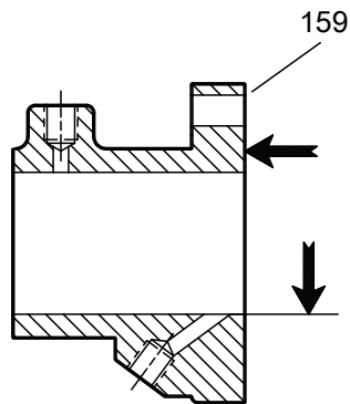
Imagen 50: Contraplato 3198
