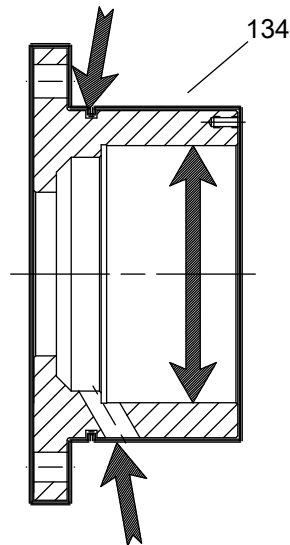
Imagen 54: Porta-rodamientos LTI
