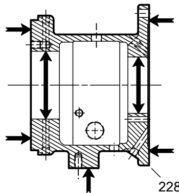
Imagen 41: Ubicaciones de inspección de la superficie exterior
