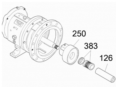
Imagen 35: Quite el asiento estacionario y la cámara de sellado
