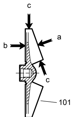
Imagen 39: Áreas para inspeccionar el desgaste en el impulsor 3196.
