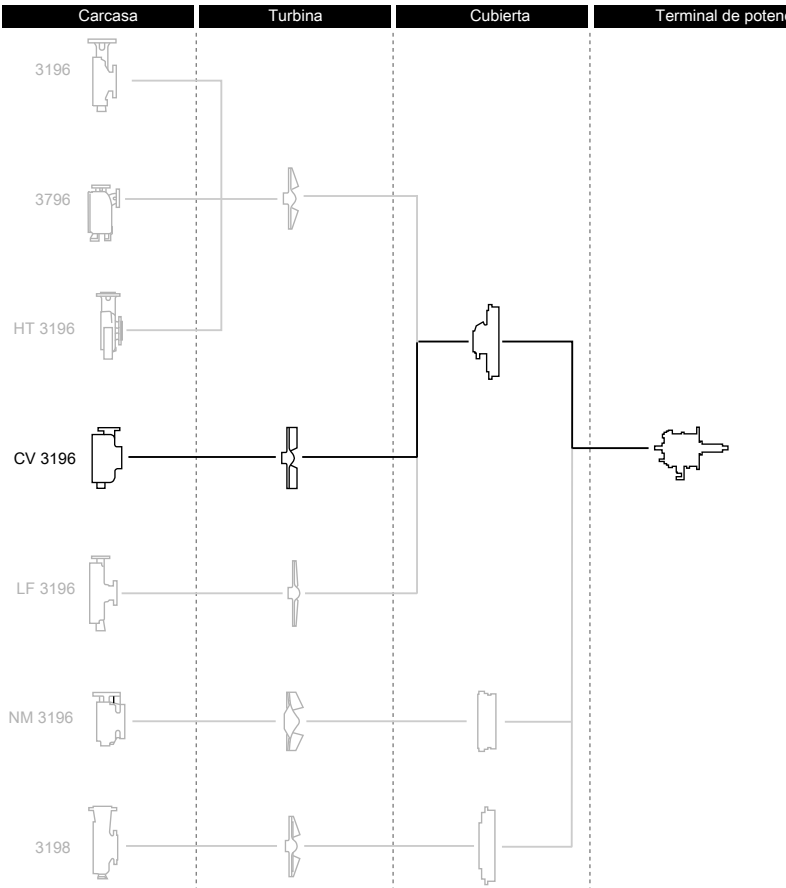
Imagen 12: Descripción de las piezas del modelo CV 3196
