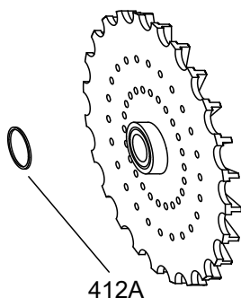
Imagen 30: Junta tórica para el modelo LF 3196
