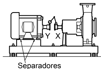
Imagen 25: Ejemplo de alineación vertical incorrecta (vista lateral)
