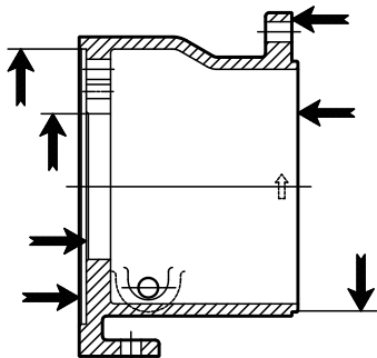
Imagen 43: Ubicaciones de inspección del adaptador de cara C
