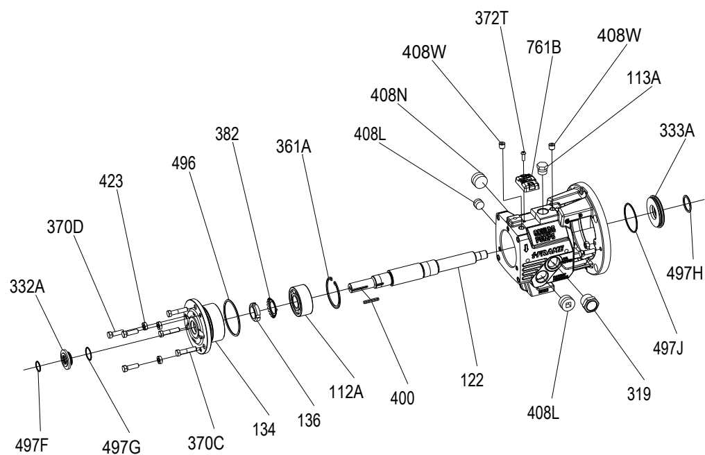
Imagen 63: Vista detallada de la caja de rodillos STi
