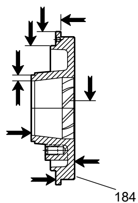
Imagen 47: TaperBore™ Plus
