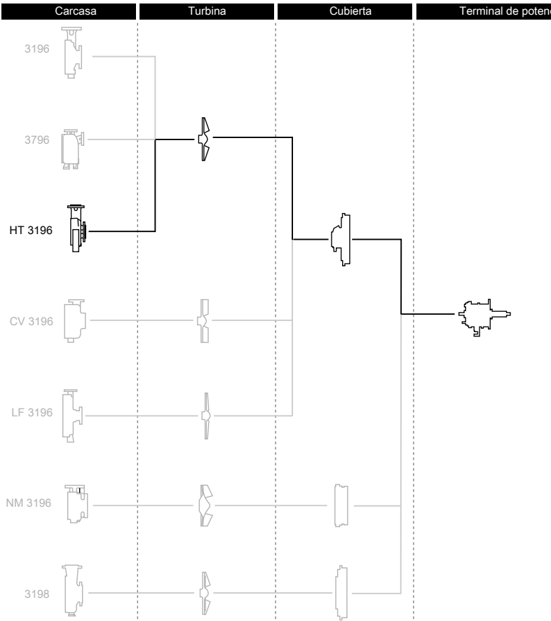
Imagen 14: Descripción de las piezas del modelo HT 3196
