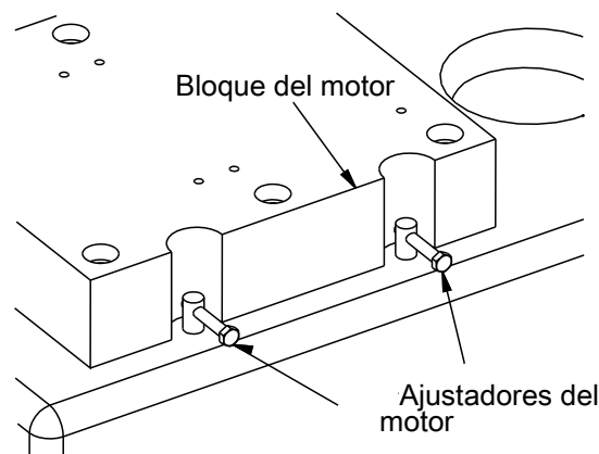
Imagen 68: Sistema de montaje de motores Polyshield Polyadjust
