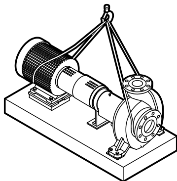
Imagen 2: Ejemplo de un método de elevación adecuado
