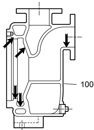
Imagen 38: Carcasa 3796
