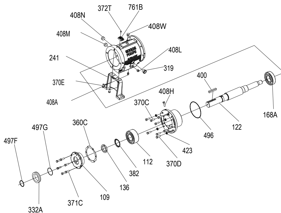
Imagen 66: Vista detallada de la caja de rodamientos XLT-i
