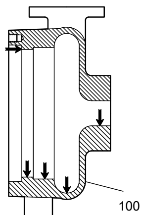
Imagen 36: Carcasas 3196, HT 3196, LF 3196, NM 3196 y 3198
