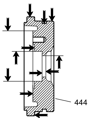
Imagen 47: TaperBore™ Plus
