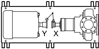
Imagen 26: Ejemplo de alineación horizontal incorrecta (vista superior)
