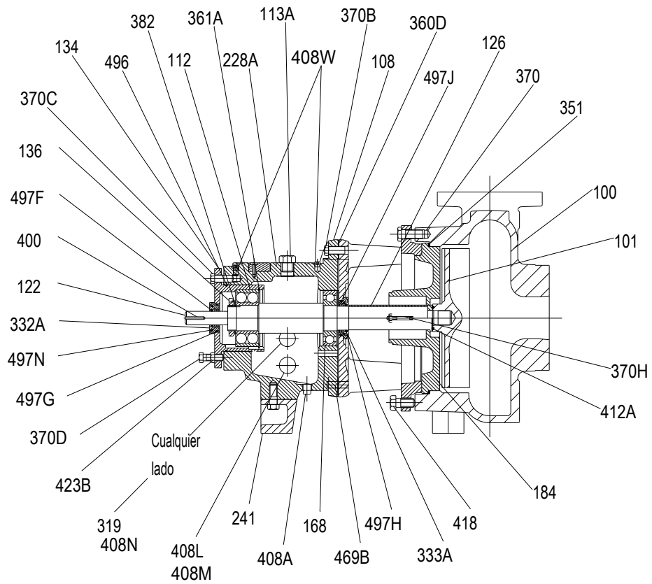
Imagen 57: Plano de la sección transversal del modelo CV 3196
