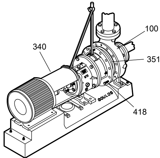
Imagen 27: Ejemplo de un adaptador de cara C (340)
