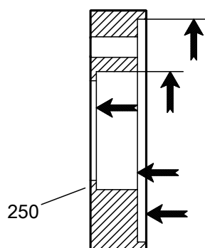
Imagen 48: Contraplato NM 3196
