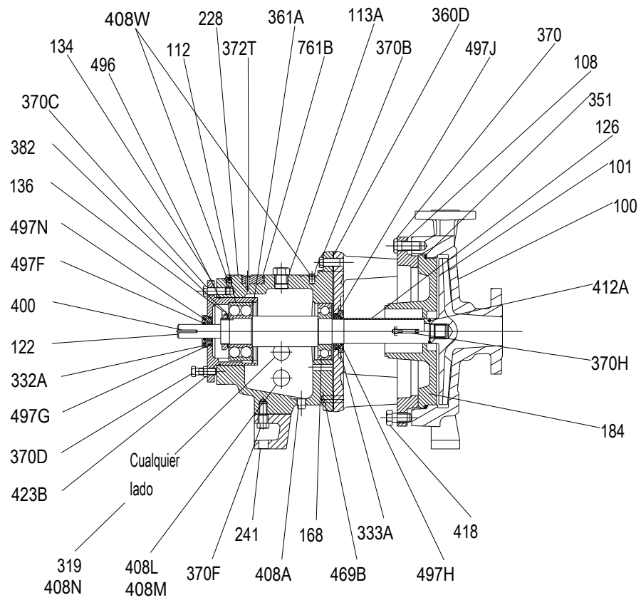
Imagen 59: Plano de la sección transversal del modelo LF-3196
