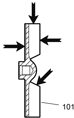
Imagen 40: Áreas para inspeccionar el desgaste en el impulsor CV 3196.
