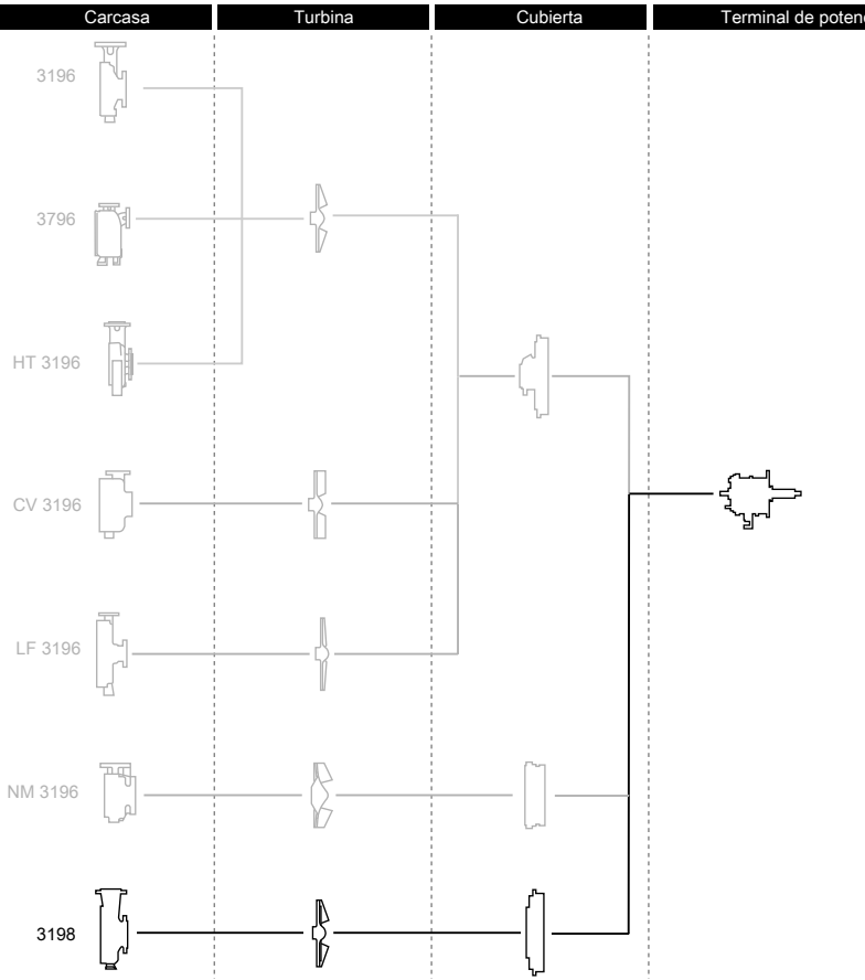
Imagen 8: Descripción de las piezas del modelo 3198
