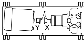
Imagen 24: Ejemplo de alineación horizontal incorrecta (vista superior)
