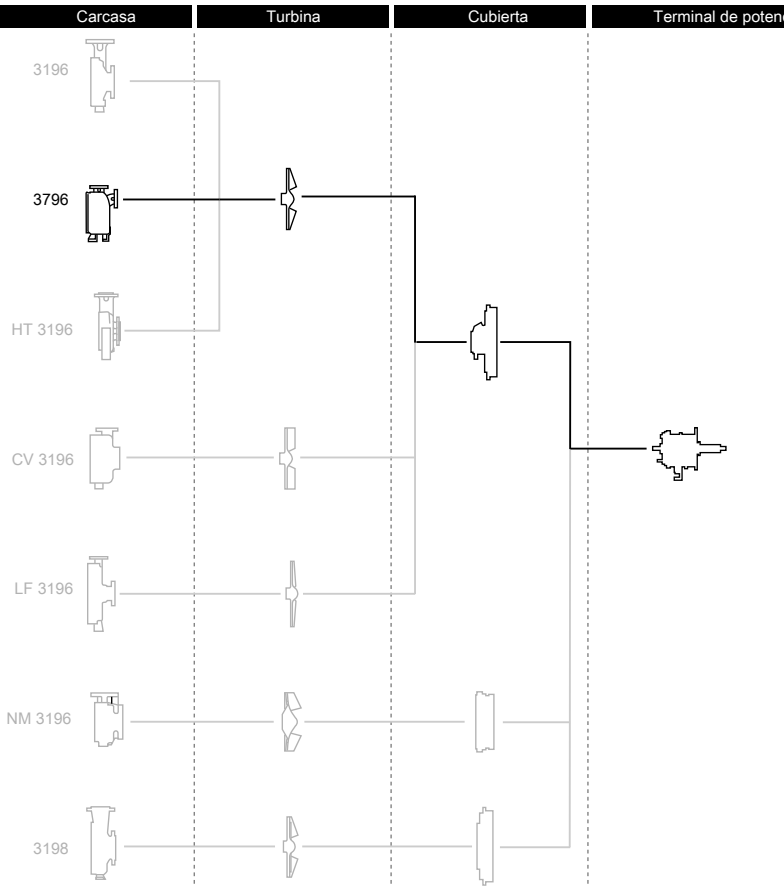
Imagen 10: Descripción de las piezas del modelo 3796
