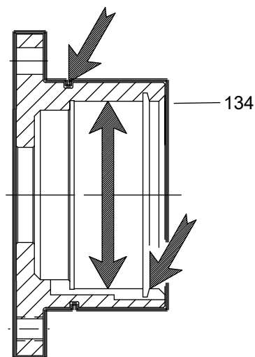
Imagen 53: Porta-rodamientos STi y MTi
