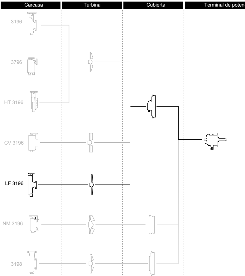
Imagen 16: Descripción de las piezas del modelo LF 3196
