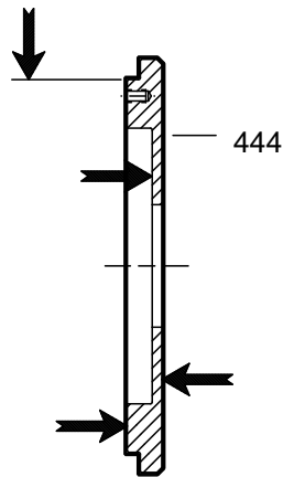
Imagen 45: Cubierta de la prensaestopas
