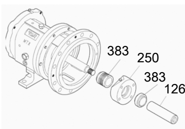
Imagen 34: Quite el asiento estacionario y el casquillo
