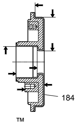
Imagen 52: 3198 BigBore™
