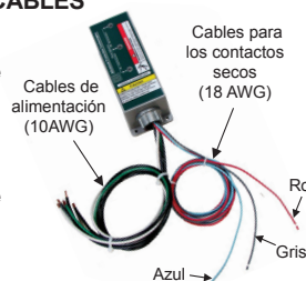
Figura 5 CABLES
