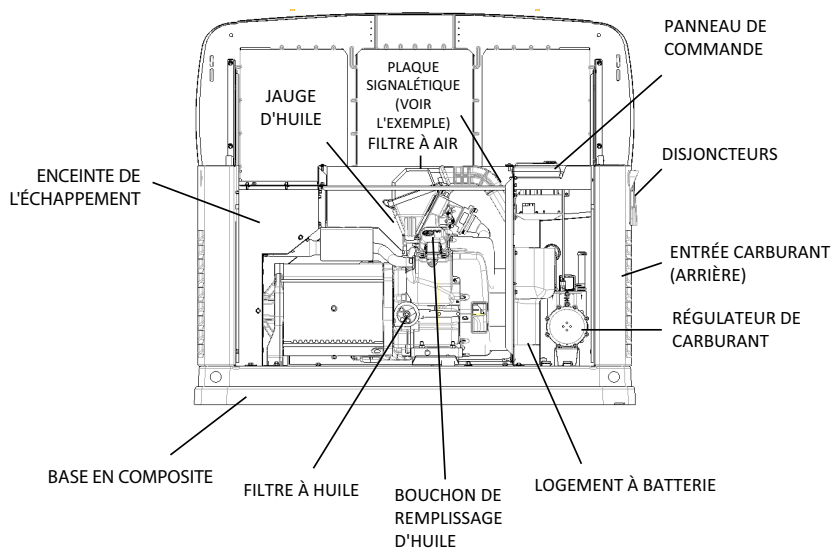
Figure 2-1 : Moteur GH-410, appareil de 8 kW
