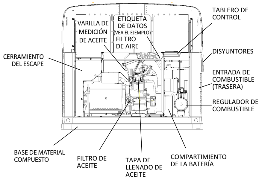
Figura 2-2: Unidad GH-530 motor de 11 kW
