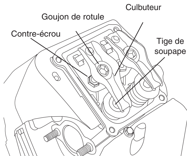
Figure 4-4 : Réglage du jeu des soupapes
