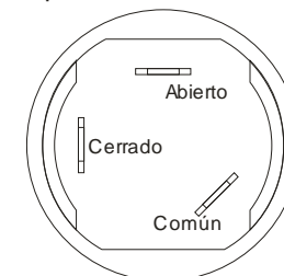
Vista posterior de la cerradura
