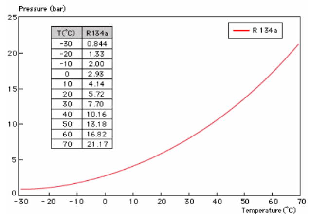
GRÁFICO PRESIÓN/TEMPERATURA
