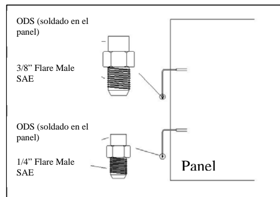
Fig. 4 Detalle de las conexiones del panel
