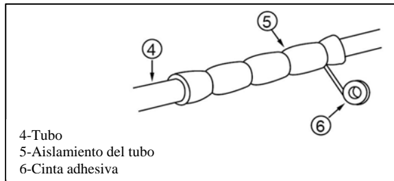
Fig. 21 Aislamiento de las conexiones
