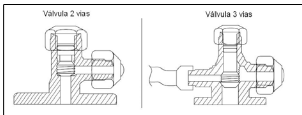
Fig. 27 Válvulas cerradas (2 y 3 vías)
