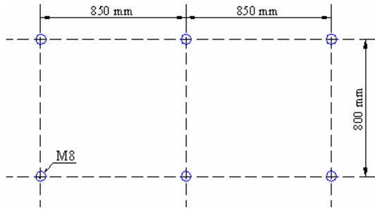
Fig. 13 Esquema de perforaciones en el panel
