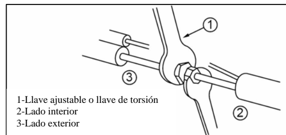
Fig. 20 Ajuste de las conexiones con llaves
