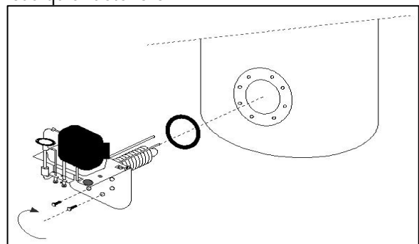
Fig. 15 Acoplamiento del Bloque al Termoacumulador
