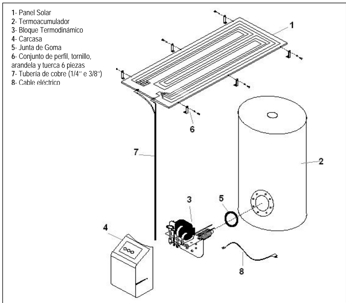
Fig. 2 Vista completa de los componentes del equipamiento
