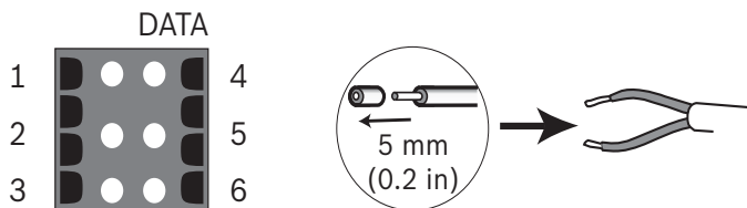
Figura 5.6 Patillas del conector de datos
