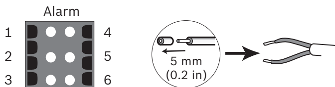
Figura 5.3 Patillas de conectores de alarma y relé
