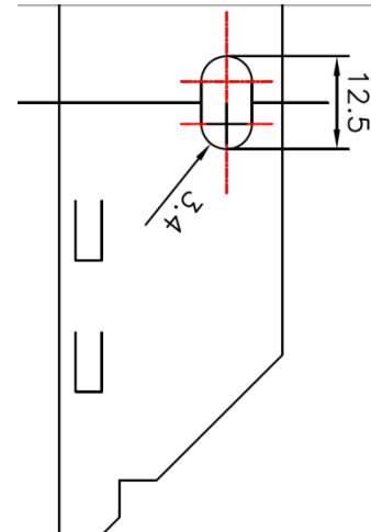
Detalle de uno de los orificios de anclaje (mm)
