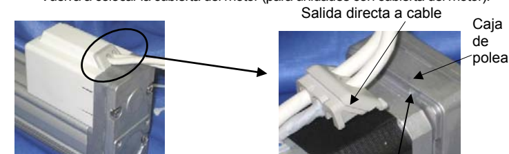
La pestaña de la salida directa a cable se inserta en el orificio de la caja de polea.
