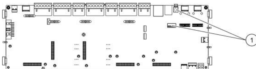
Figura 21: Los conectores USB de la PCB de la central
