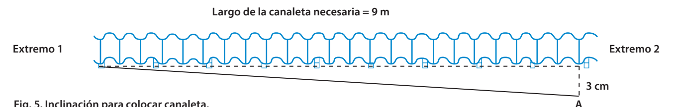
Fig. 5. Inclinación para colocar canaleta.
