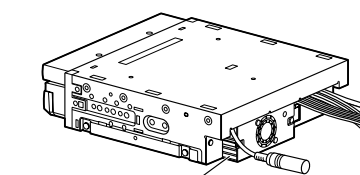
Heat sink / Sumidero térmico
