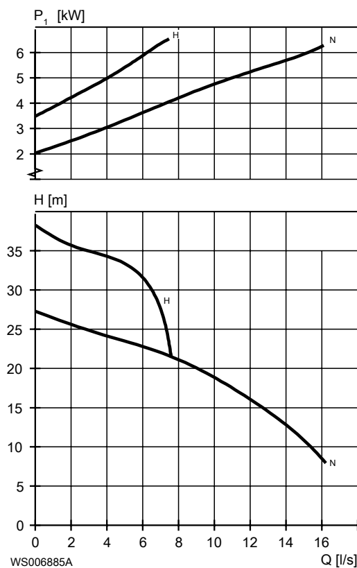
Imagen 12: 50 Hz
