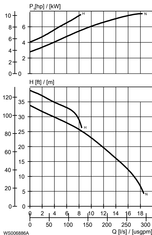
Imagen 13: 60 Hz
