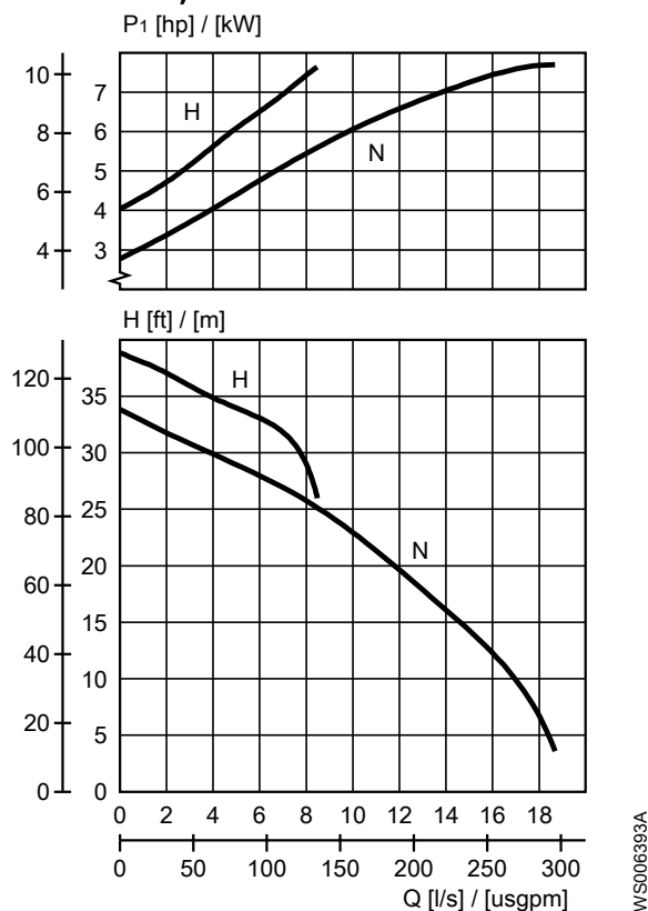
Imagen 12: 50 Hz
