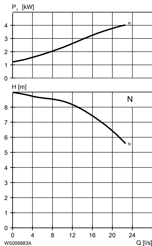
Imagen 11: 50 Hz
