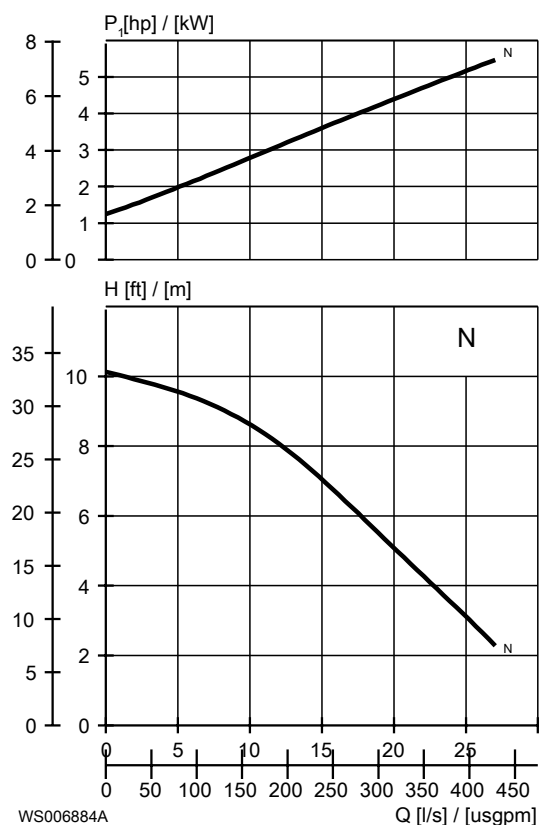
Imagen 12: 60 Hz
