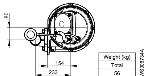
Imagen 10: H, DN 75 mm
