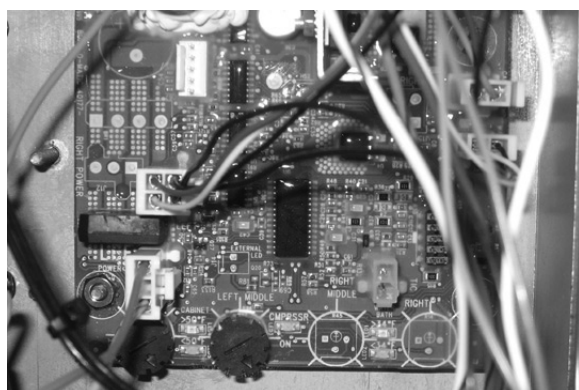
FIG 14A LED de Temperatura-JDF-2S (Modelos Anteriores)
