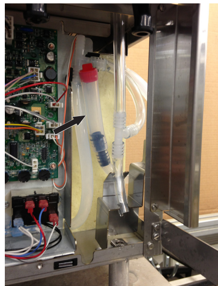
FIG 4 Tubo flexible de llenado inicial - JDF-4S
