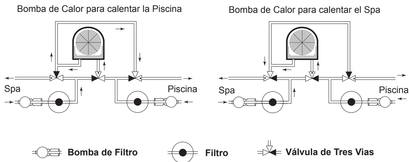
Figura 3. Sistema de Filtrado Compartido
