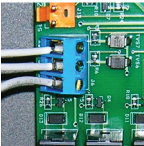
Figura 15a. Conexión Pool-Off-Spa Remota (Conexión de 3 Cables)
