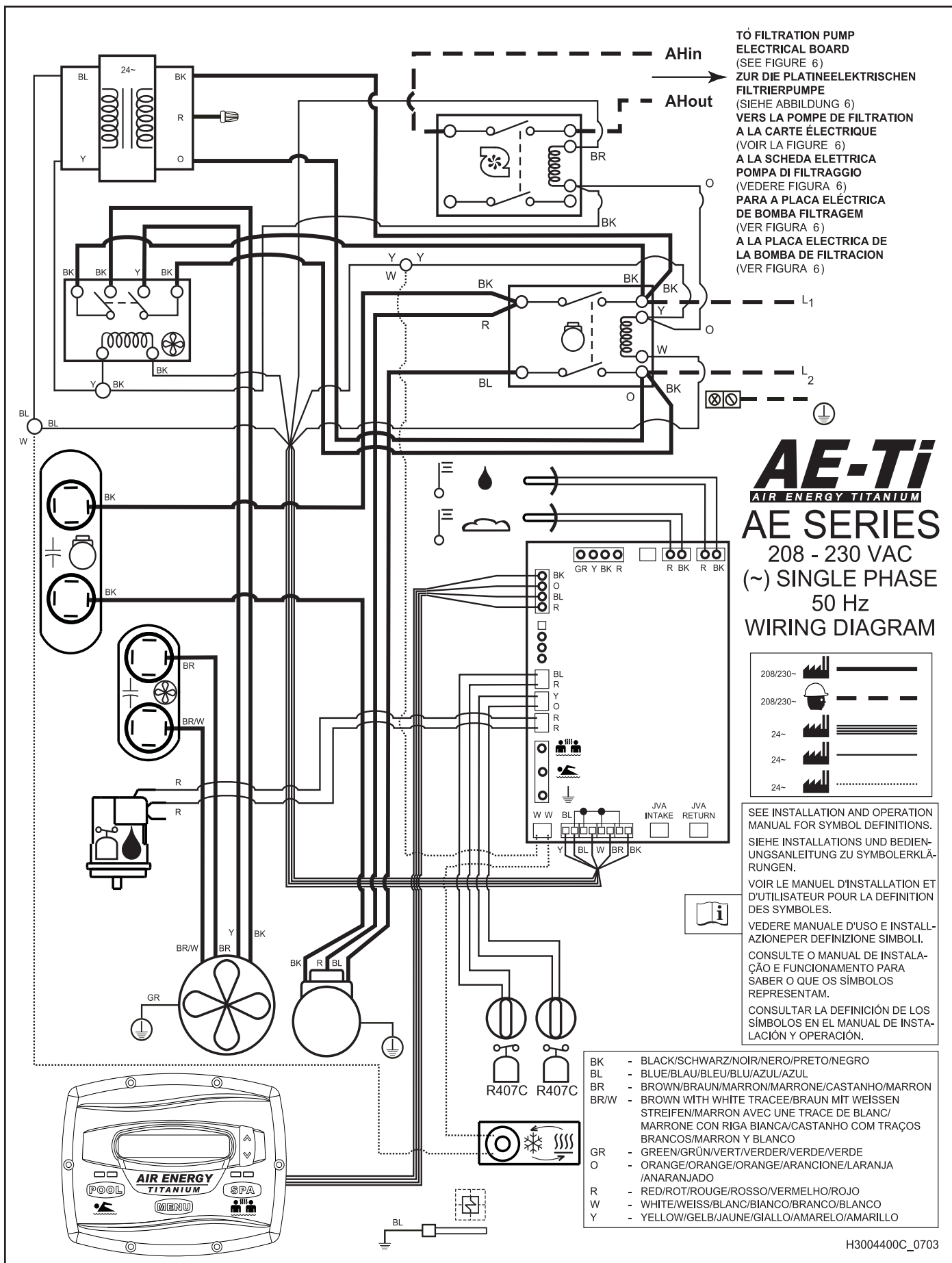
Figura 10. Diagrama de Cableado de Alimentación de Energía Monofásica del Modelo AE-Ti
