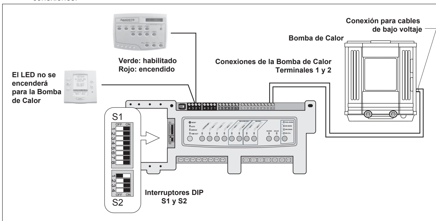
Figura 16. Cableado AquaLink RS a Bomba de Calor
