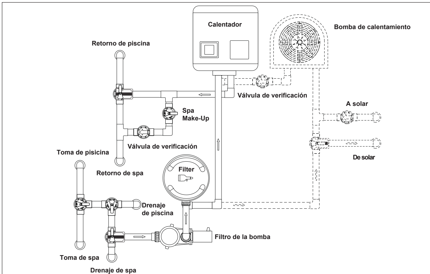
Figura 5. Plomería para Combinación de Sistemas de Calentamiento
