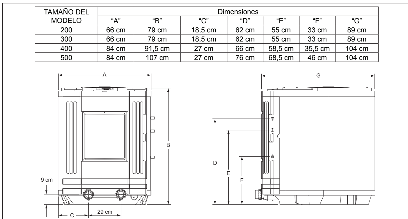
Figura 1. Dimensiones de la Bomba de Calor AE-Ti
