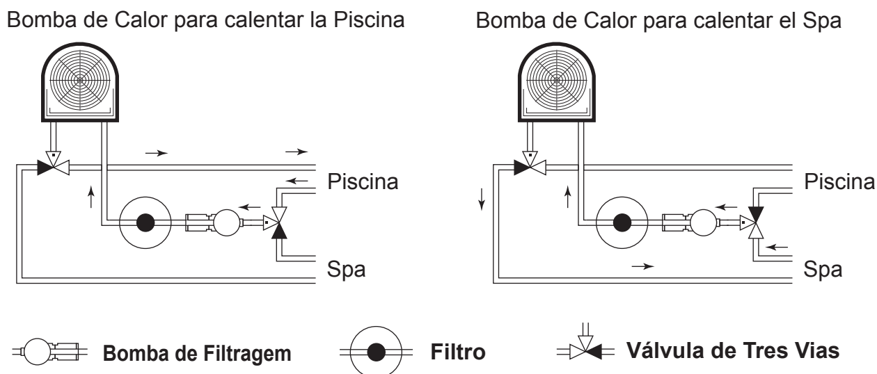
Figura 4. Sistema de Bomba Dual (Sistemas de Filtrado Independientes que Comparten una Bomba de Calor)
