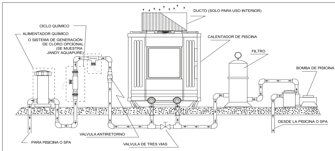
Figura 2. Diagrama de Plomería Básica
