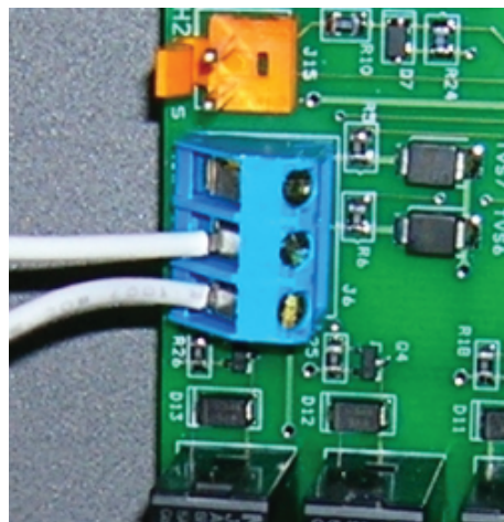
Figura 15b. Conexión AquaLink RS o TERMOSTATO REMOTO (Conexión de 2 Cables)
