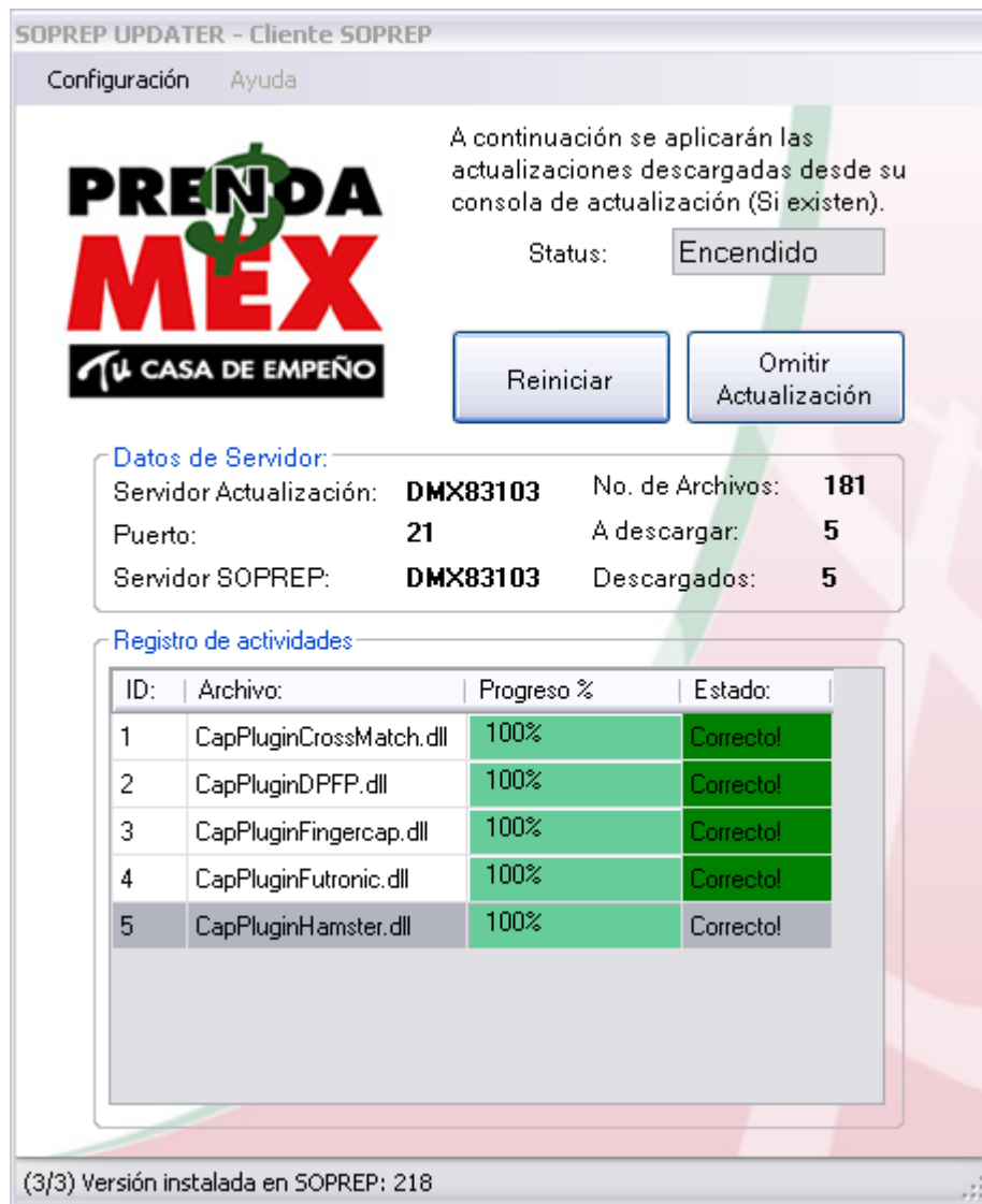
Fig.9 Actualizador cliente durante descargas.
