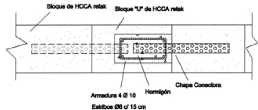
Anclaje de R.V. en encadenado
