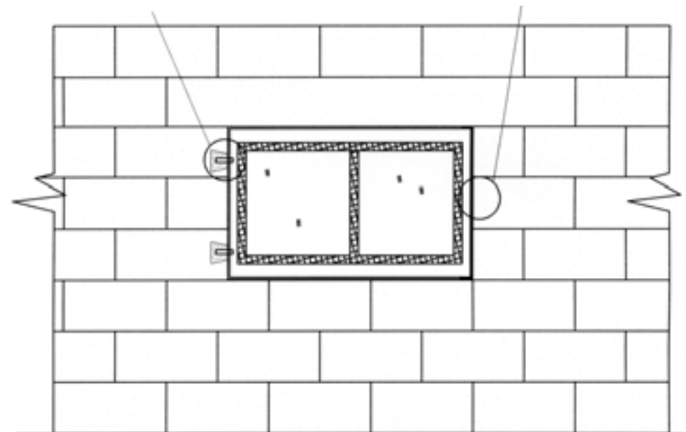
Fijación tradicional con mortero de cemento 1:3
