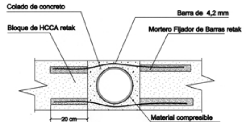
VISTA A-A
