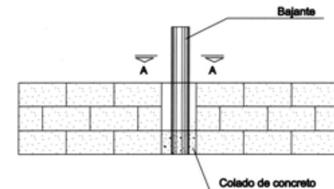
VISTA A-A
