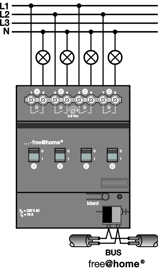
Fig. 3: Conexión eléctrica
