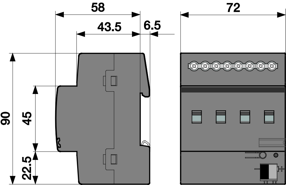
Fig. 2: Dimensiones
