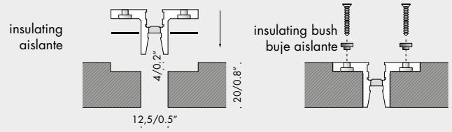
on wood mounting example cremagliera B ejemplo de montaje cremagliera B en la madera
