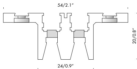
1:1 section cremagliera C sección 1:1 cremagliera C
