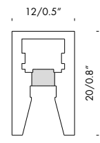
1:1 section cremagliera A sección 1:1 cremagliera A
