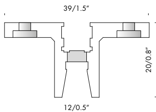
1:1 section cremagliera B sección 1:1 cremagliera B
