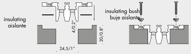
on wood mounting example cremagliera C ejemplo de montaje cremagliera C en la madera
