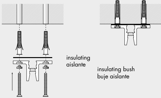
wall mounting example cremagliera C ejemplo de montaje cremagliera C en pared
