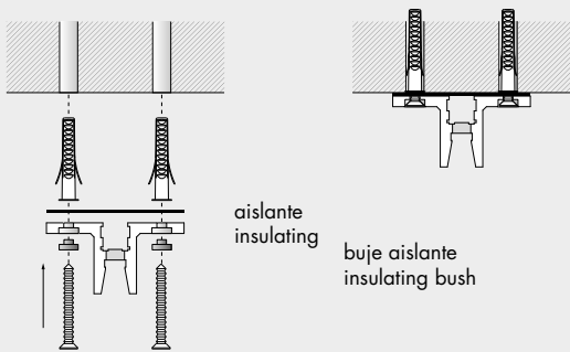
ejemplo de montaje cremagliera C en pared wall mounting example cremagliera C
