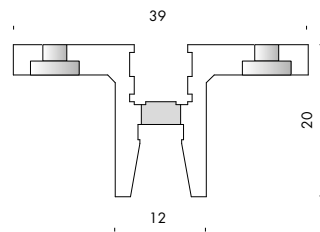
sección 1:1 cremagliera B 1:1 section cremagliera B
