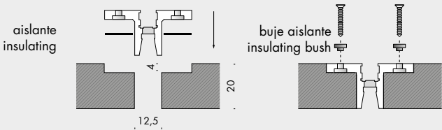
ejemplo de montaje cremagliera B en la madera on wood mounting example cremagliera B
