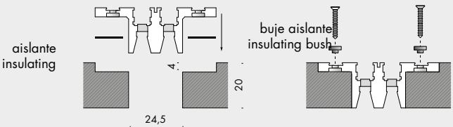
ejemplo de montaje cremagliera C en la madera on wood mounting example cremagliera C
