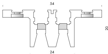
sección 1:1 cremagliera C 1:1 section cremagliera C
