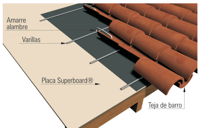
fig. 4.7.3 Base para techo cubierta en teja de barro
