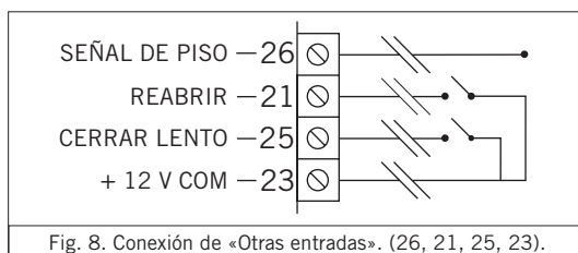
Fig. 8. Conexión de «Otras entradas». (26, 21, 25, 23).
