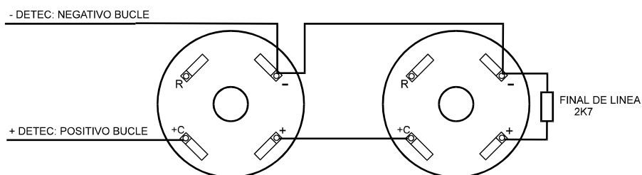
Fig.: 2 Conexión del bucle de detectores.
