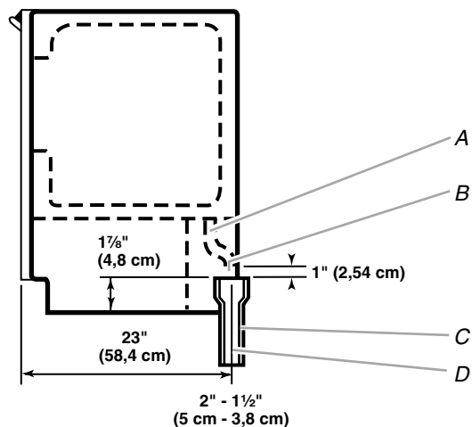
A. Manguera de desagüe B. Espacio de aire de 1" (2,54 cm) C. Reductor de desagüe de PVC D. El centro del desagüe debe estar a 23" (58,4 cm) desde el frente de la puerta, con o sin el panel de \frac{3}{4} " (1,91 cm) en la puerta. El desagüe debe también estar centrado de izquierda a derecha ( 7\frac{5}{16} " [18,56 cm] de cada lado de la fábrica de hielo).
