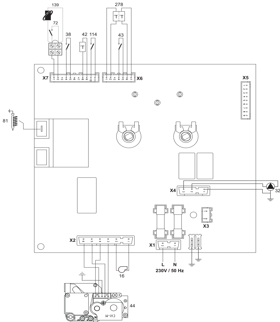
fig. 21 - Esquema eléctrico
