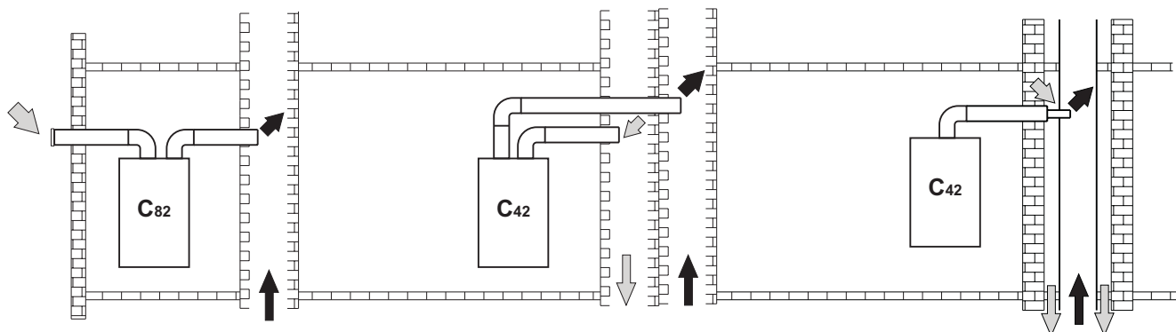
fig. 13 - Ejemplos de conexión a chimeneas (⇨ = aire / ⇨ = humos)
