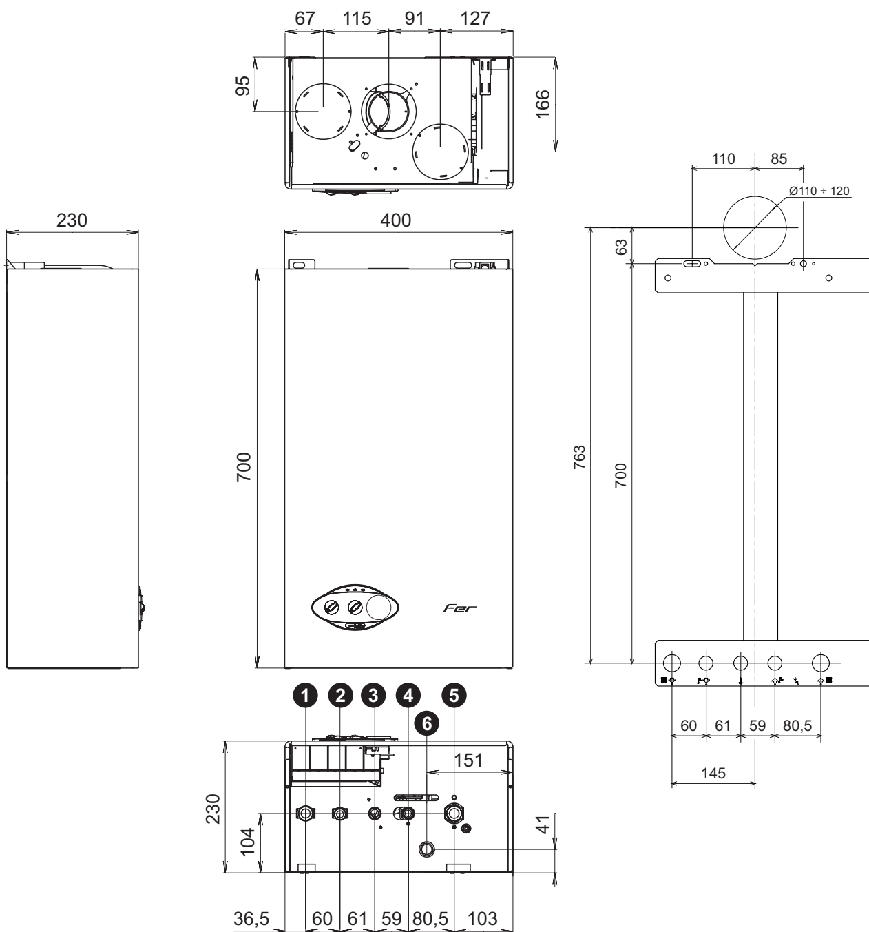
fig. 18 - Dimensioni e attacchi
