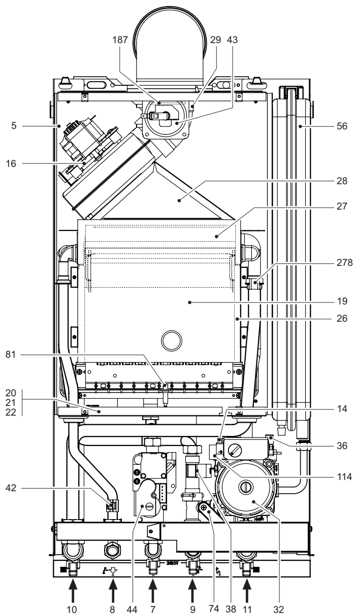
fig. 19 - Vista generale
