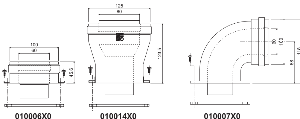
fig. 10 - Accessori di partenza per condotti coassiali
