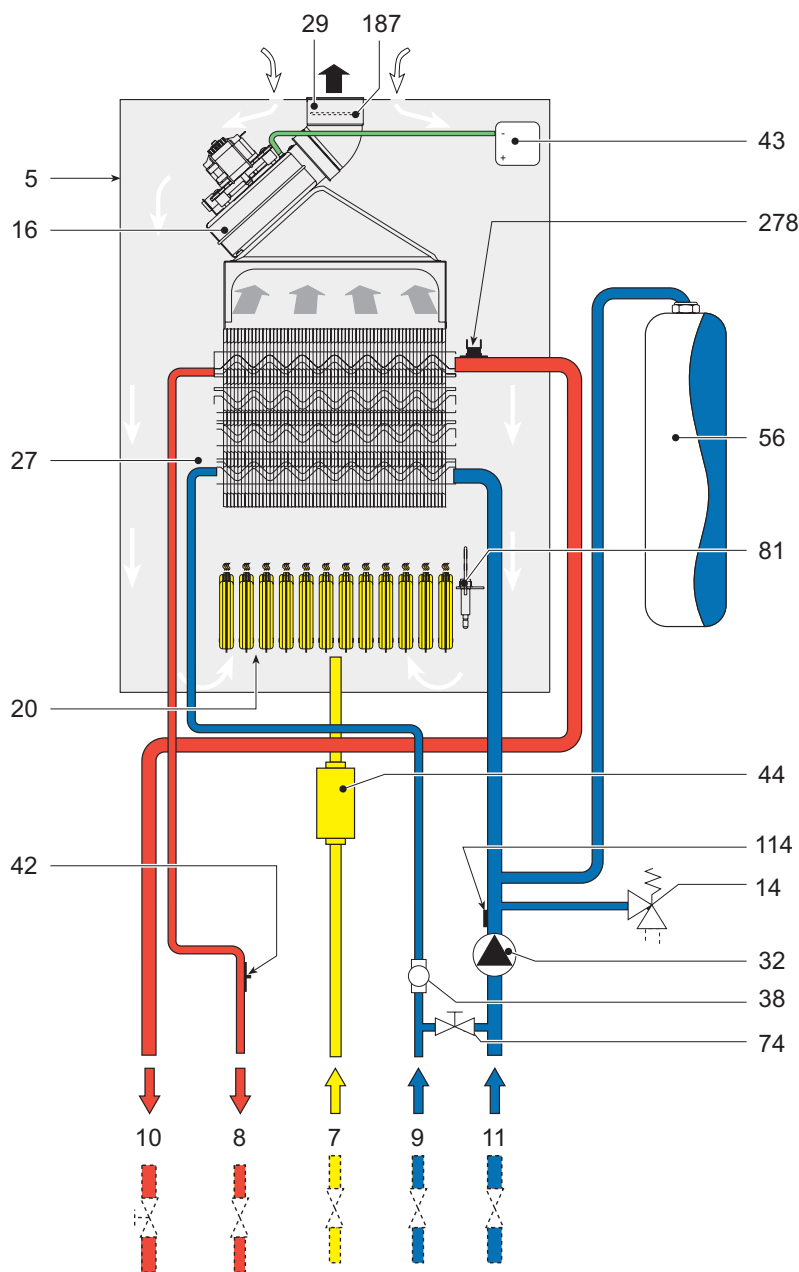
fig. 20 - Circuito hidráulico
