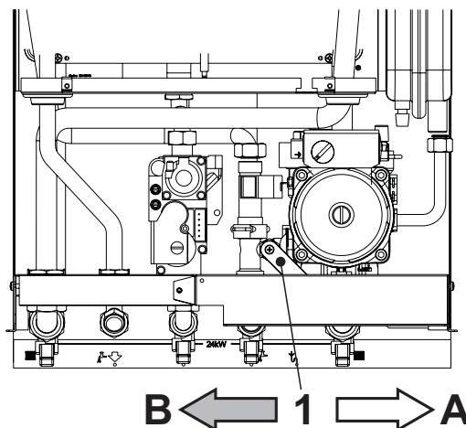
fig. 4 - Llave de llenado
