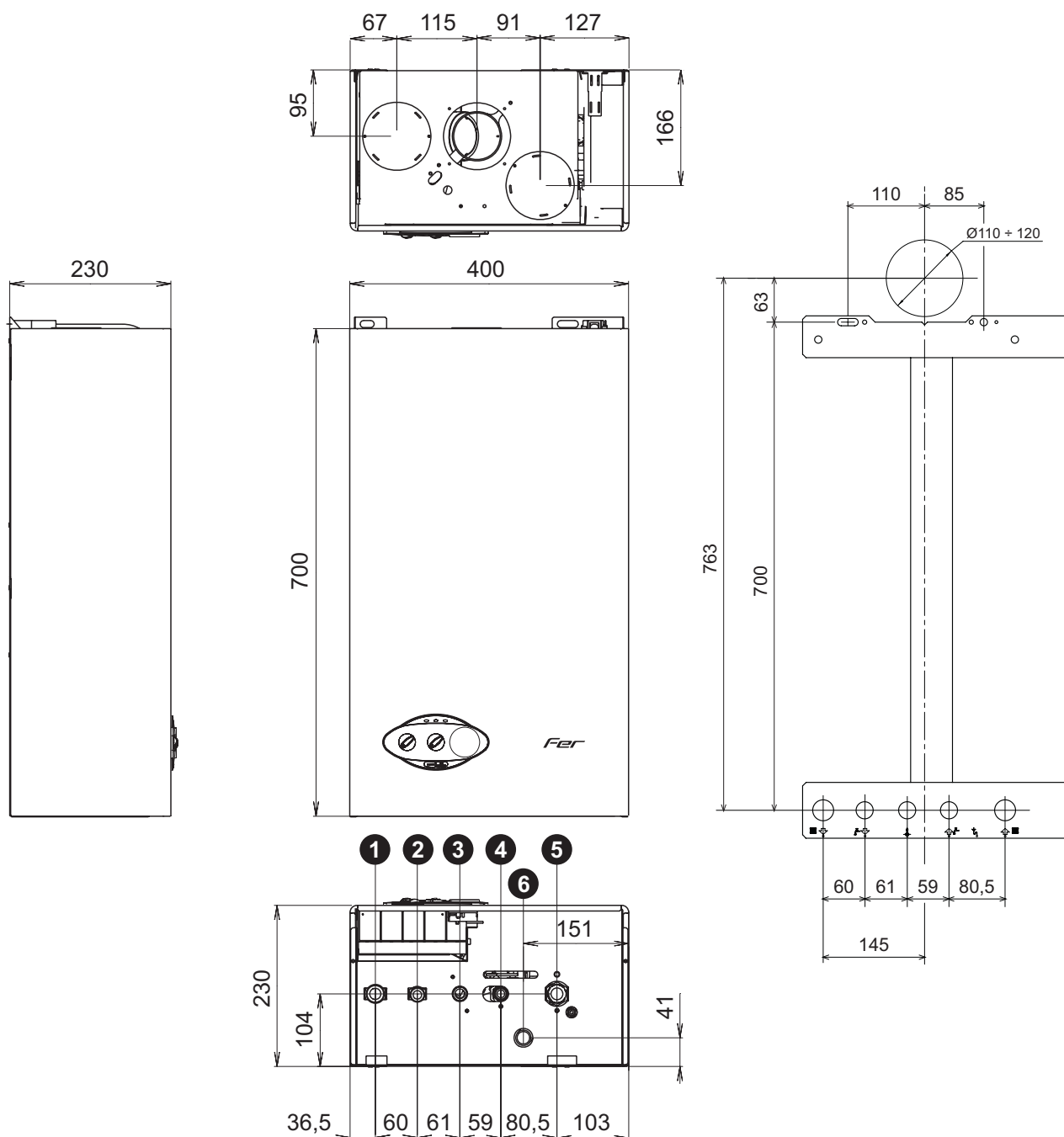
fig. 18 - Dimensiones y conexiones
