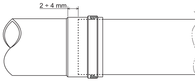
fig. 7 - Dilatación
