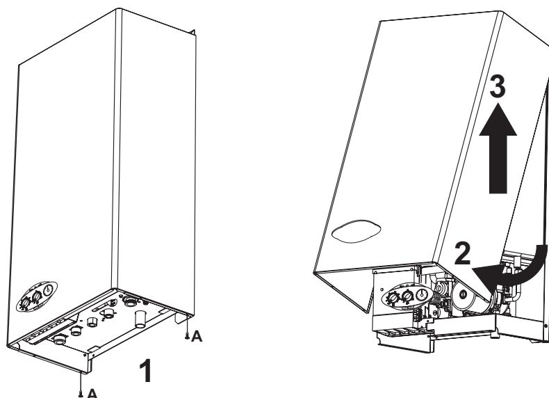
fig. 16 - Apertura mantello
