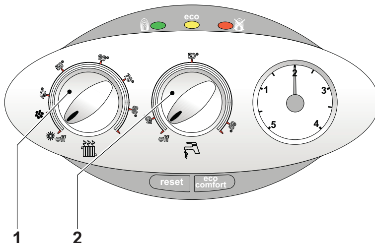
fig. 2 - Caldaia spenta
