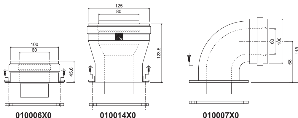
fig. 10 - Accesorios iniciales para conductos coaxiales
