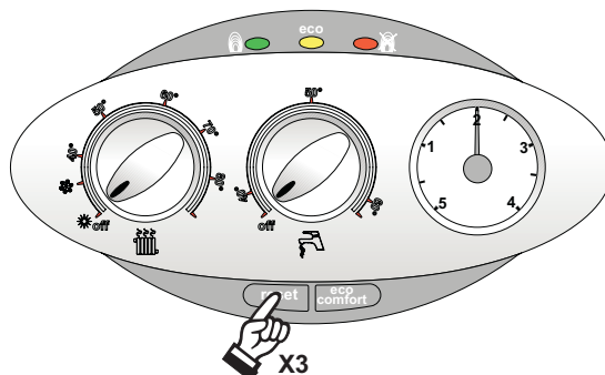
fig. 14 - Modalità TEST
