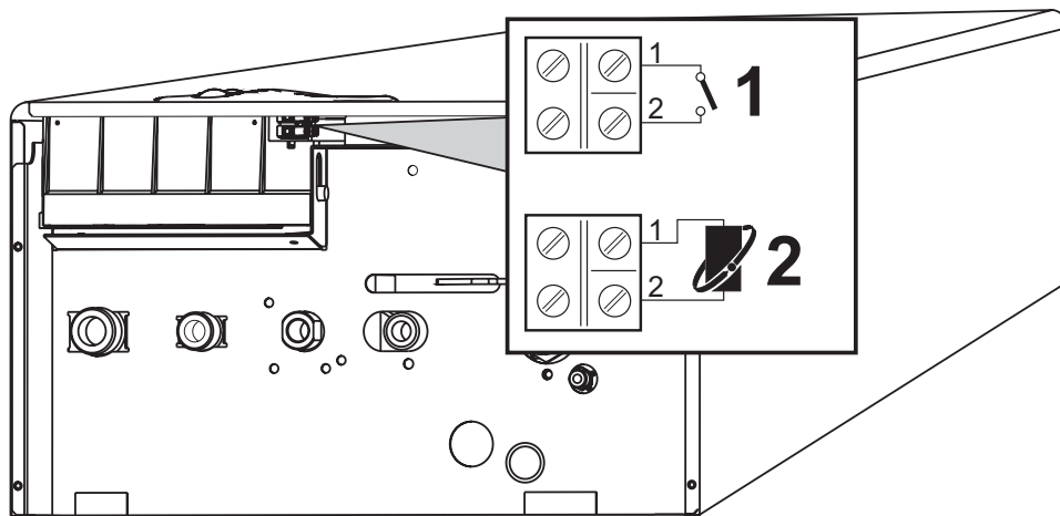
fig. 6 - Accesso alla morsettiera
