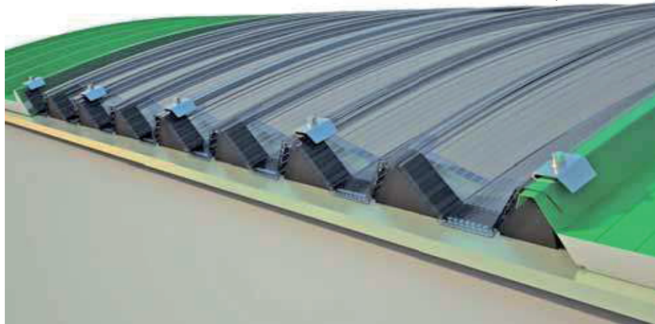
DETALLE DE LA FIJACIÓN detalle de la fijación de las placas en las correas.
