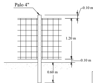
DETALLE DE ANCLAJE DE PARANTES (ESC. 1:60)
