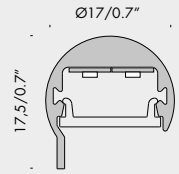
1:1 section tubino s sección 1:1 tubino s
