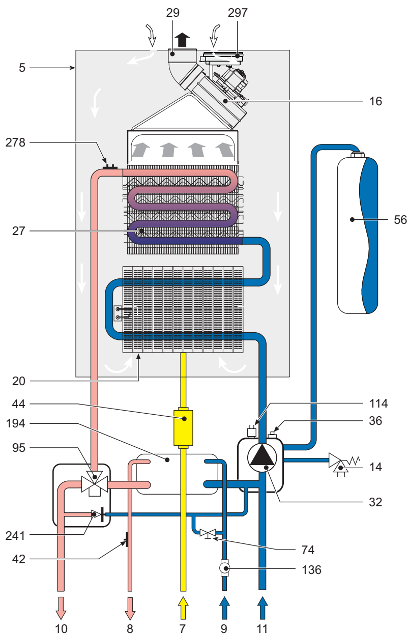
fig. 27 - Circuitul hidraulic
