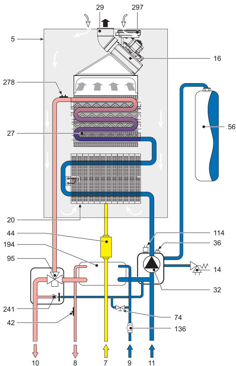
fig. 27 - Circuito hidráulico
