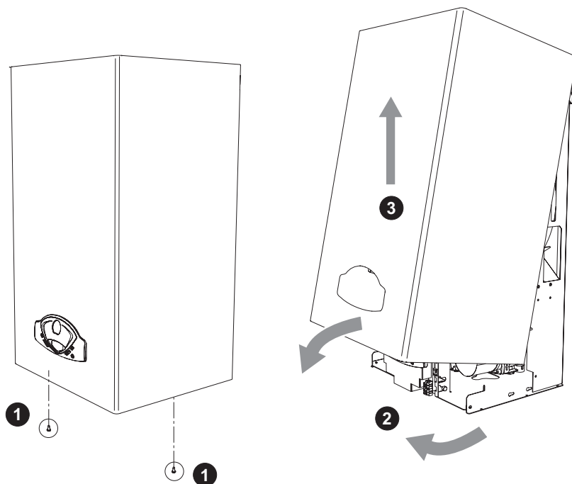
рис. 23 - Демонтаж кожуха
