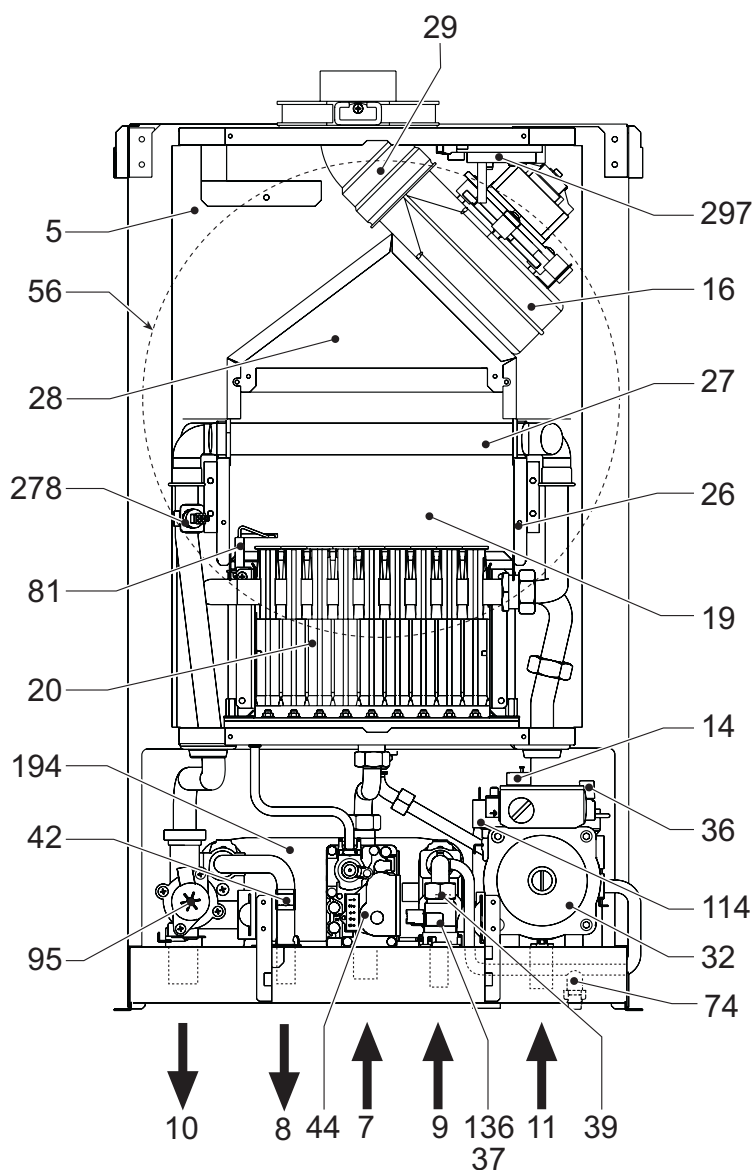
fig. 26 - Vista generale
