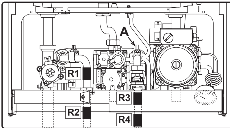
fig. 17 - Poziționarea încălzitoarelor și a termostatlui antiîngheț
