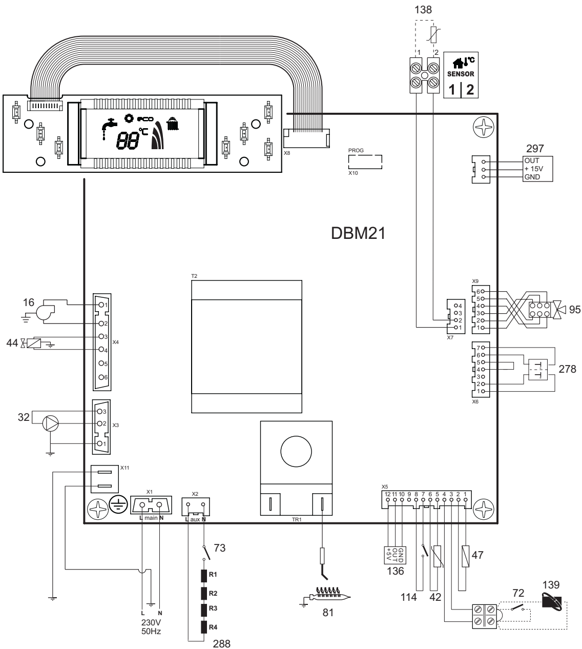
рис. 28 - Электрическая схема
