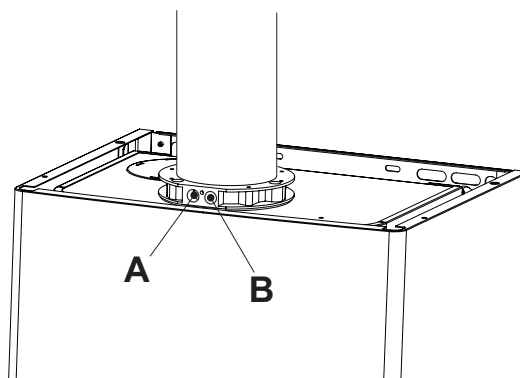
fig. 24 - Analizarea combustiei
