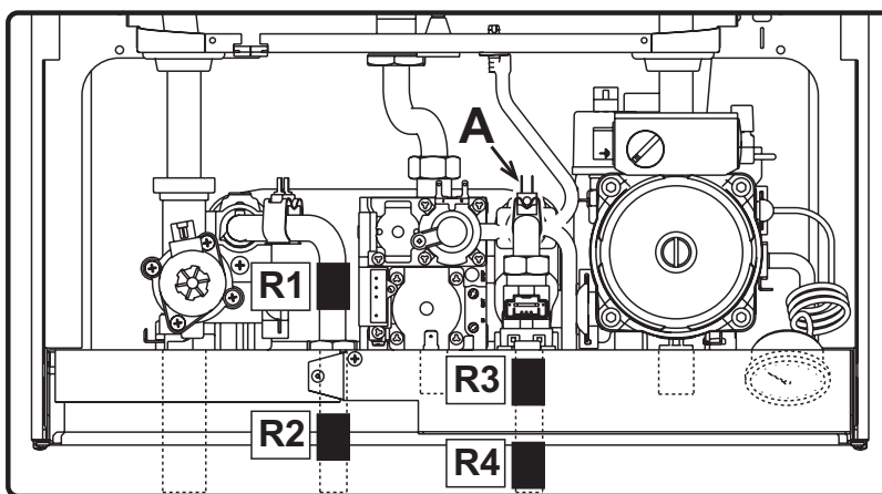
fig. 17 - Posizionamento riscaldatori e termostato antigelo
