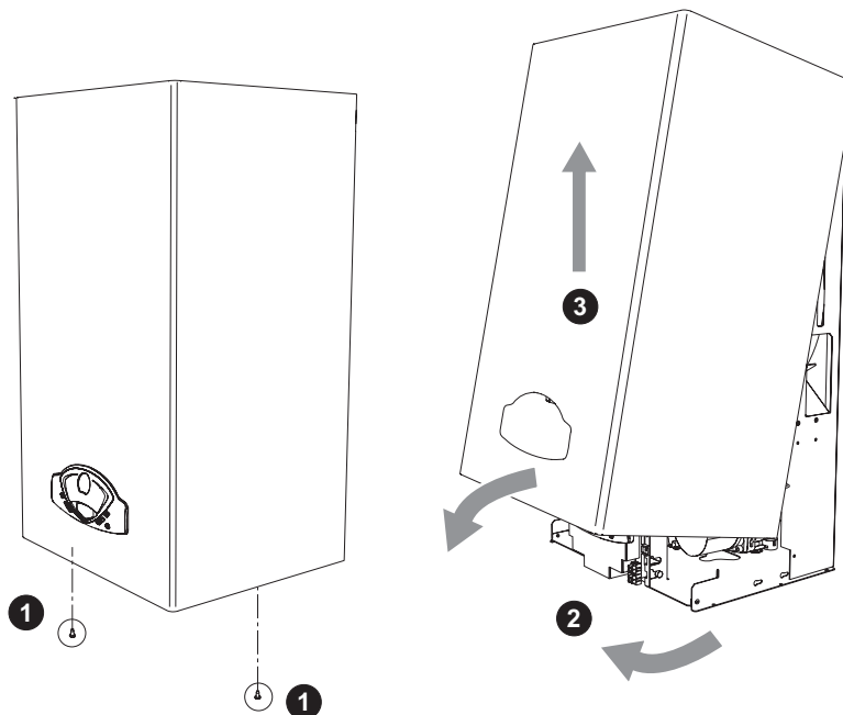
fig. 23 - Deschiderea carcasei
