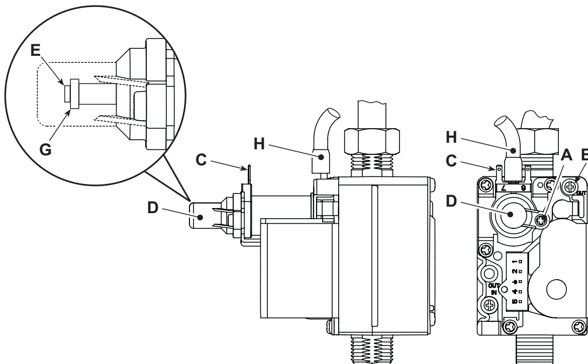
рис. 22 - Газовый клапан
