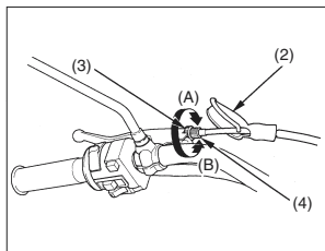
(2) Guardapolvo (3) Contratuercas (4) Ajustador (A) Aumenta el juego (B) Disminuye el juego
