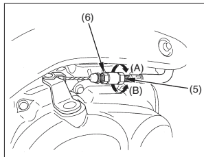
(5) Contratuercas (6) Tuerca de ajuste (A) Aumenta el juego (B) Disminuye el juego
