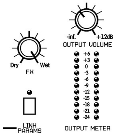
Figura 2.3: Sección maestra
