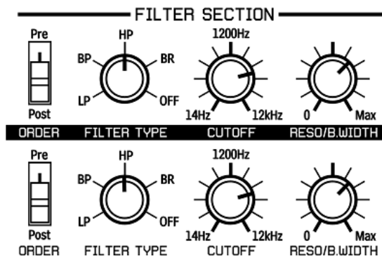
Figura 2.2: Sección del filtro dual
