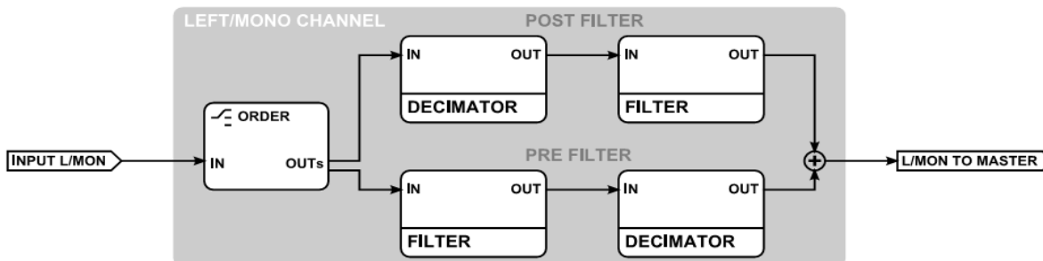
Figura 2.4: Flujo de una señal mono a través del Decimator y el Filtro
