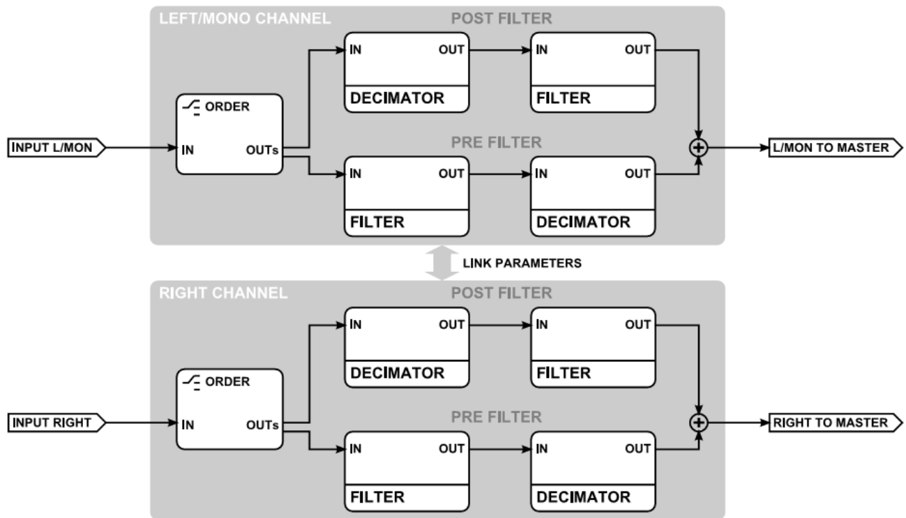
Figura 2.5: Flujo de una señal estéreo a través del Decimador y el Filtro
