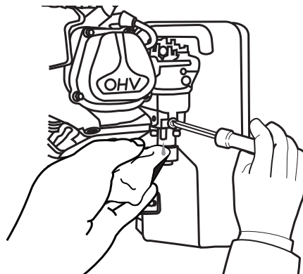
FIGURE 50: Receptáculo para drenaje de combustible
