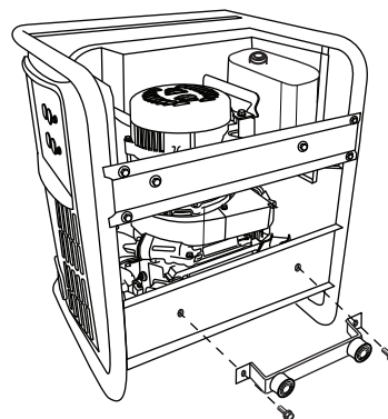
FIGURA 7: Instalación de la pata de apoyo en el generador
