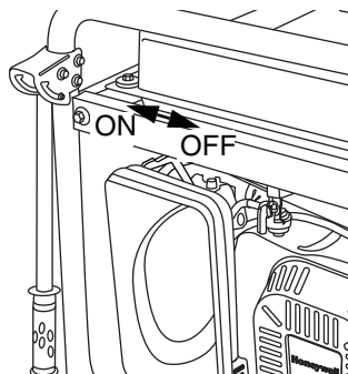
FIGURA 18: Palanca del estrangulador
