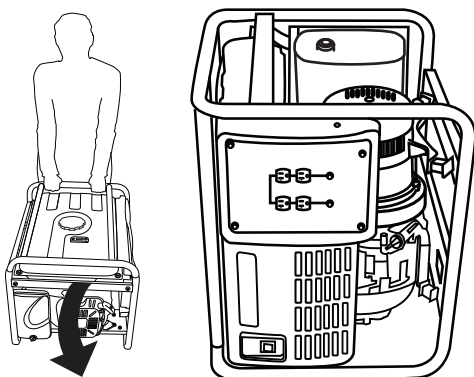
FIGURA 5: Incline hacia el lado de la cuerda de arranque del generador
