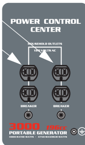
FIGURA 15: Generador portátil HW3000L
