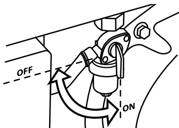
FIGURA 17: Válvula de corte de combustible — Posición ON/OFF (Encendido/Apagado)
