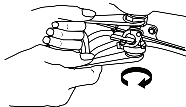
FIGURA 45: Retiro del conjunto del receptáculo para sedimentos de combustible
