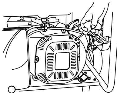
FIGURA 20: Manija del arrancador manual
