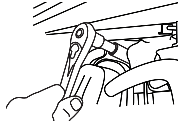
FIGURA 41: Retiro de la bujía
