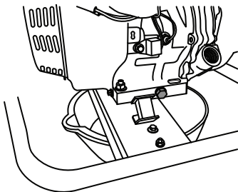
FIGURA 25: Perno de drenaje de aceite
