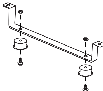
FIGURA 6: Instalación del tapones de goma en la pata de apoyo
