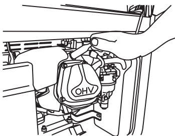
FIGURA 40: Retiro de la tapa de la bujía
