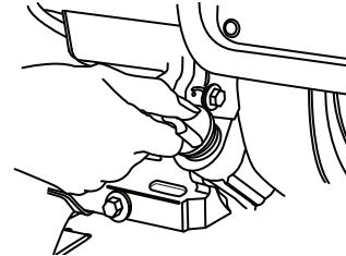
FIGURA 27: Retire la tapa para llenado de aceite
