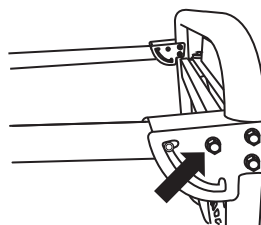
FIGURA 13: Apriete el perno de la barra de la manija
