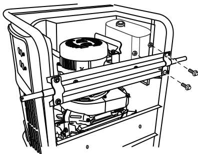
FIGURA 8: Eje de la rueda instalado en el generador
