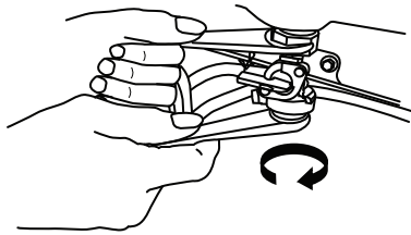
FIGURA 47: Suelte el perno para drenar el combustible
