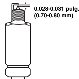
FIGURA 42: Distancia correcta entre electrodos
