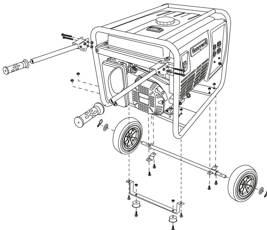
FIGURA 4: Conjunto del kit de accesorios
