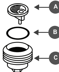
FIGURA 46: Montaje del receptáculo para sedimentos de combustible
