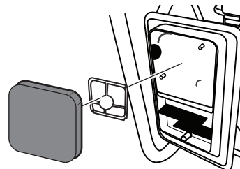
FIGURA 38: Instalación del filtro de aire - Modelo HW3000
