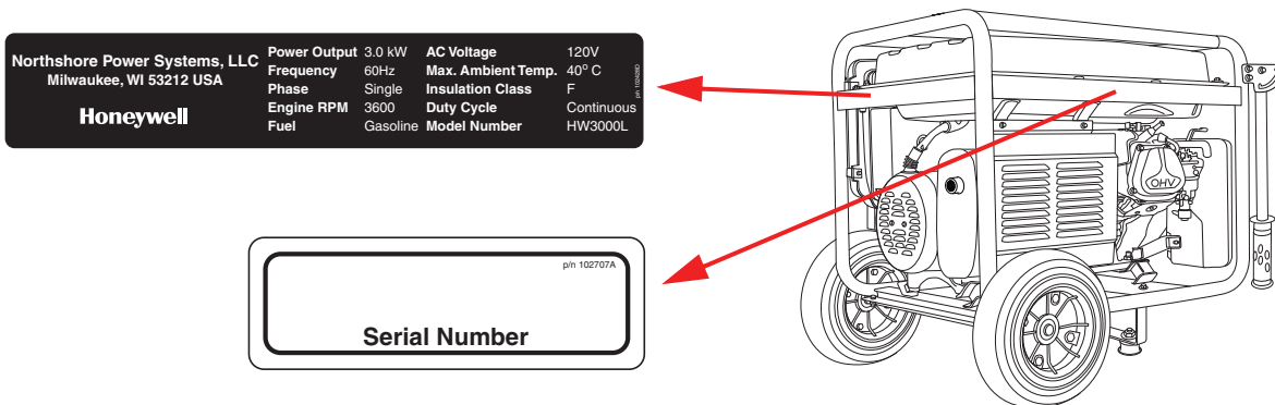
FIGURA 1: Ubicaciones de las etiquetas
