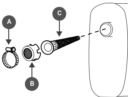
FIGURA 43: Conjunto del protector contra chispas
