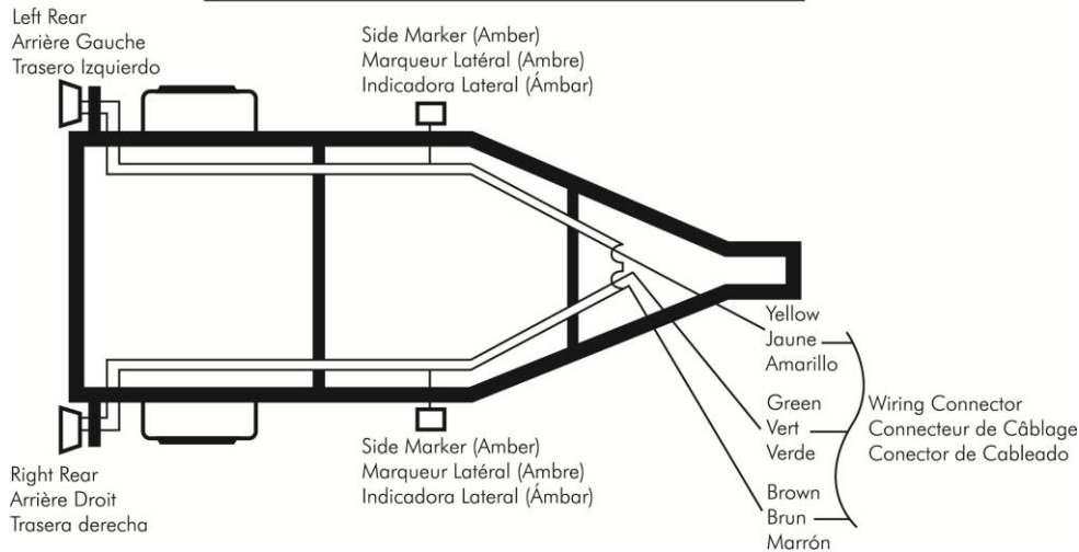
Top View of Trailer Wiring Diagram Vue de Dessus du Schéma de Câblage de la Remorque Vista Desde Arriba del Diagrama de Cableado del Remolque
