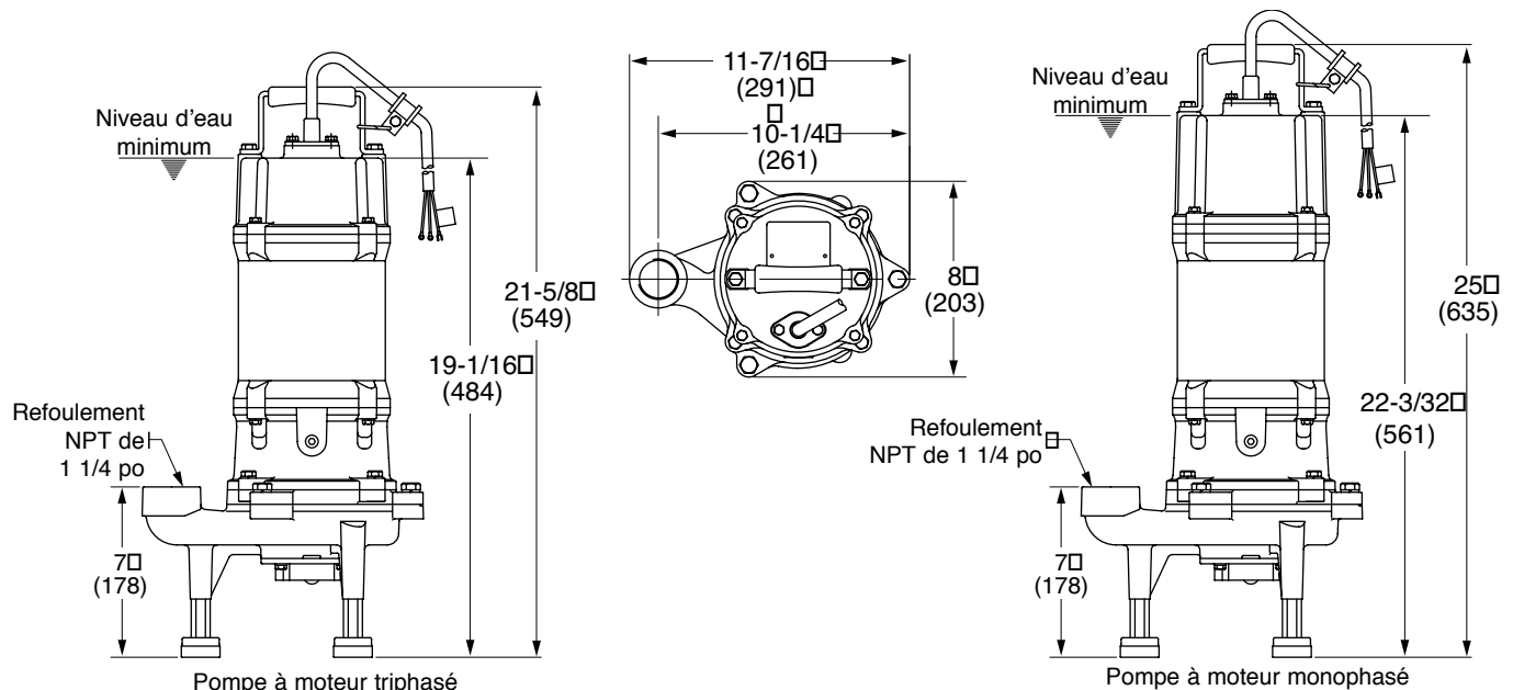
Figure 1: Dimensions en pouces (mm)
