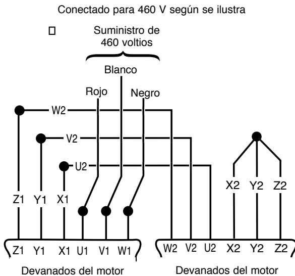
Figura 3: Conexiones de cables trifásicos de 460 Voltios
