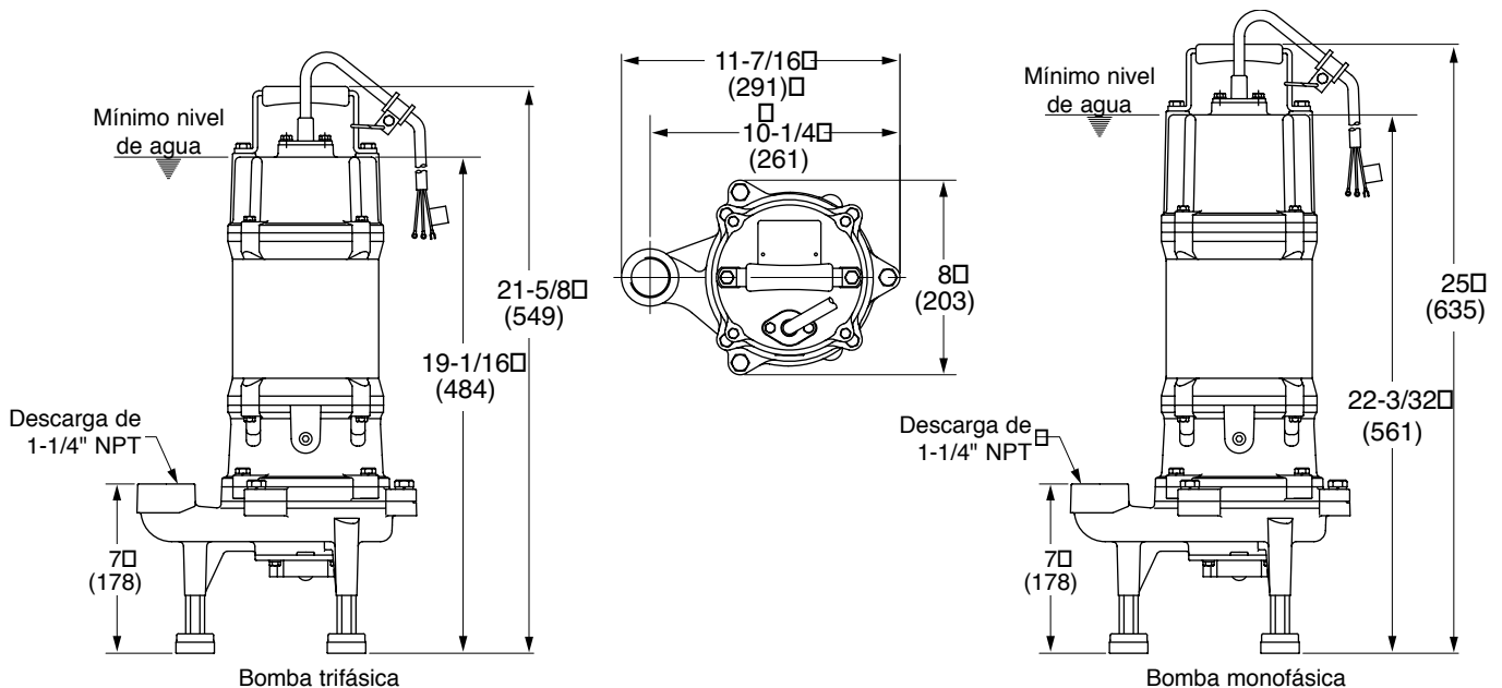
Figura 1: Dimensiones en pulgadas (mm)
