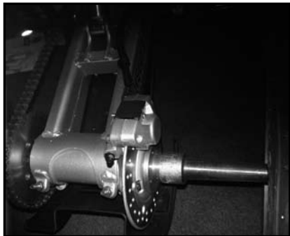
Rueda trasera con freno a disco
