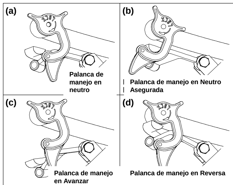
FIGURA 2 OPERACIÓN DEL CERROJO Y LA PALANCA DE MANEJO
