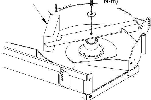
FIGURA 5 INSTALACION DEL PERNO DE LA CUCHILLA (números De serie 510,000 al 539,999)
