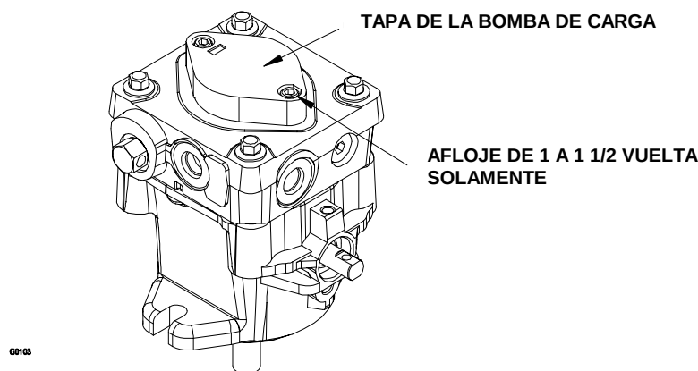
FIGURA 4 UBICACIÓN DE LA BOMBA DE CARGA
