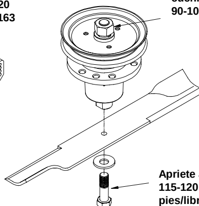
FIGURA 5 INSTALACION DEL PERNO DE LA CUCHILLA (números De serie 510,000 al 539,999)
