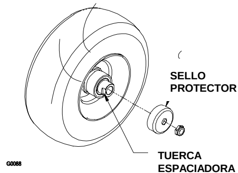
FIGURA 4 ENSAMBLE RUEDA DELANTERA
