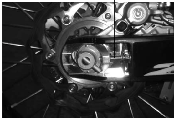
Tensor regulación
