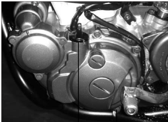
Bouchon remplissage Vis de vidange et vis de niveau
